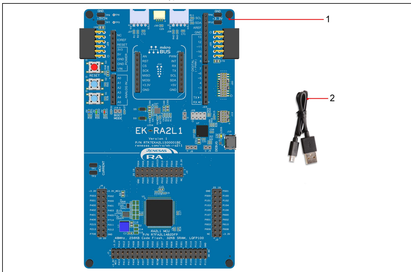
図 1 EK-RA2L1 評価キット構成
