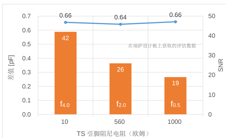
图 5-54. 阻尼电阻值和灵敏度特性
