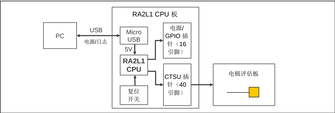
图 5-4. 评估板框图
