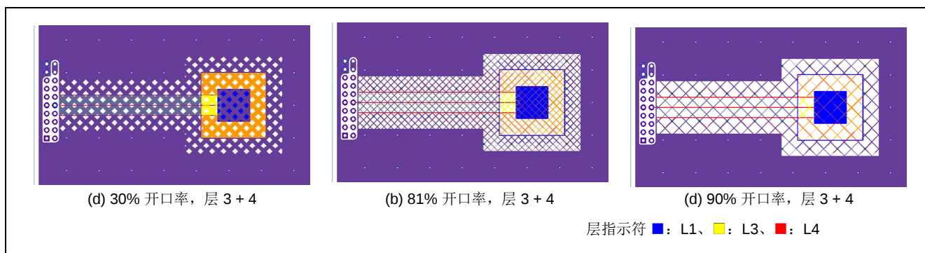
图 5-34. 评估板图案（4 层板，GND 屏蔽）
