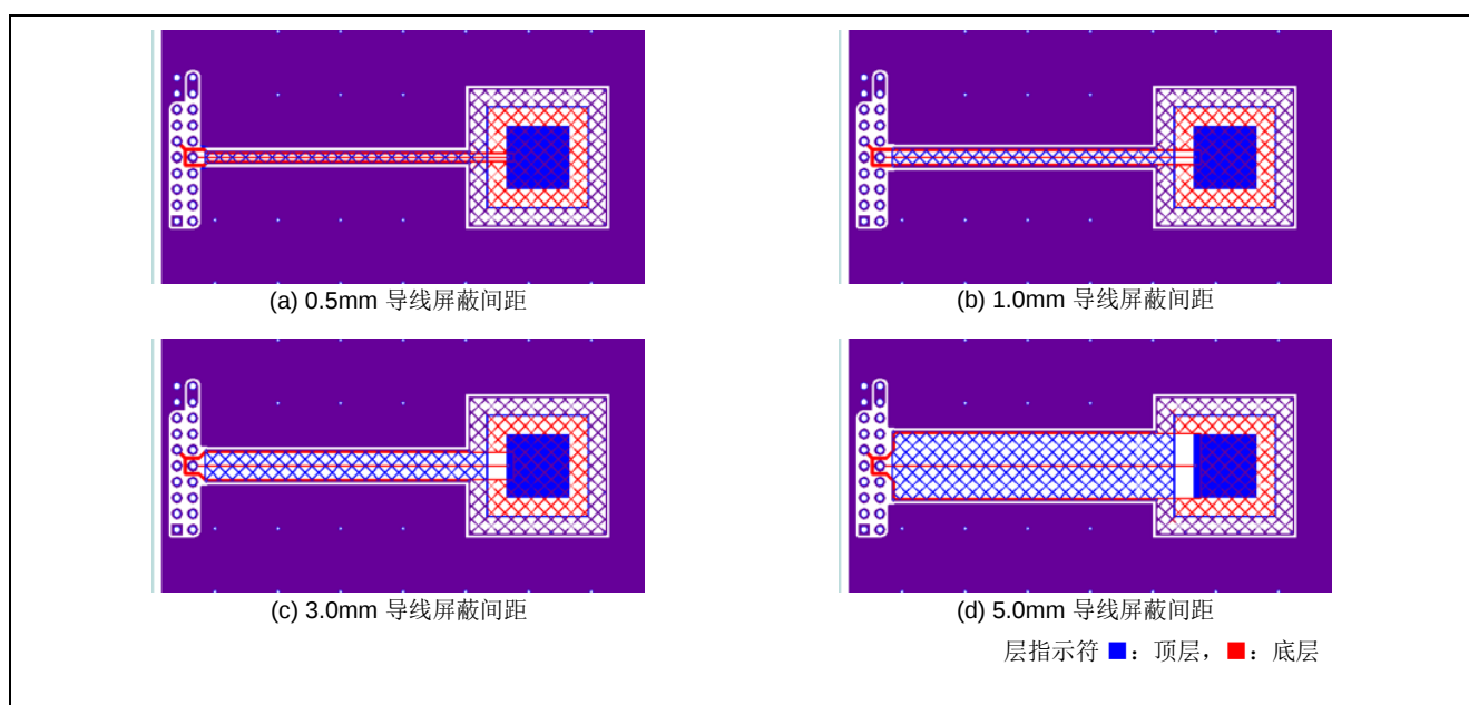
图 5-40. 评估板图案（导线与有源屏蔽间距）
