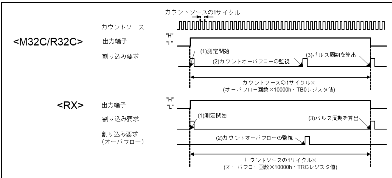
図 2.4 パルス幅測定例
