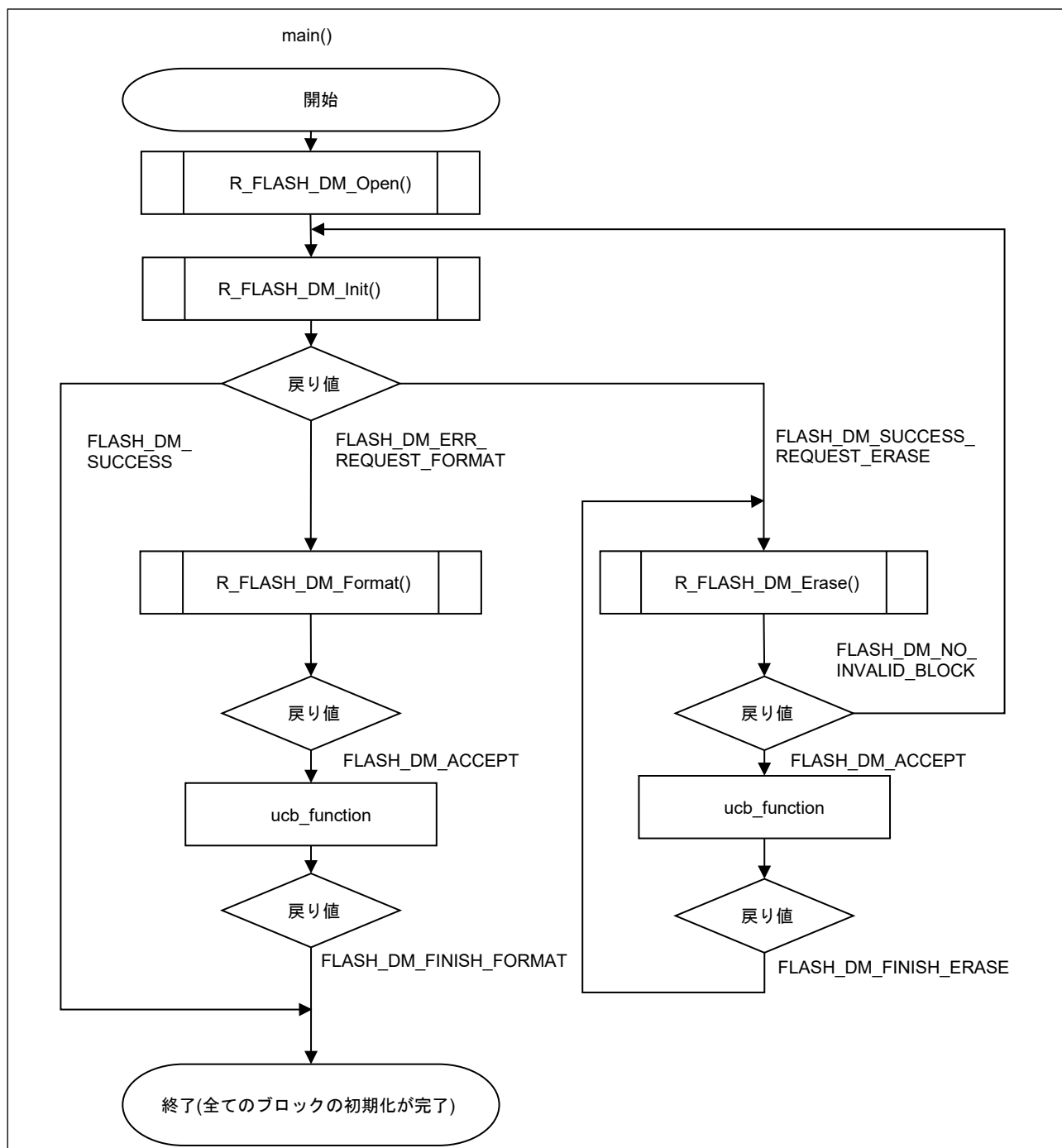
図 1-3 R_FLASH_DM_Init()後の処理例(フラッシュタイプ1)
