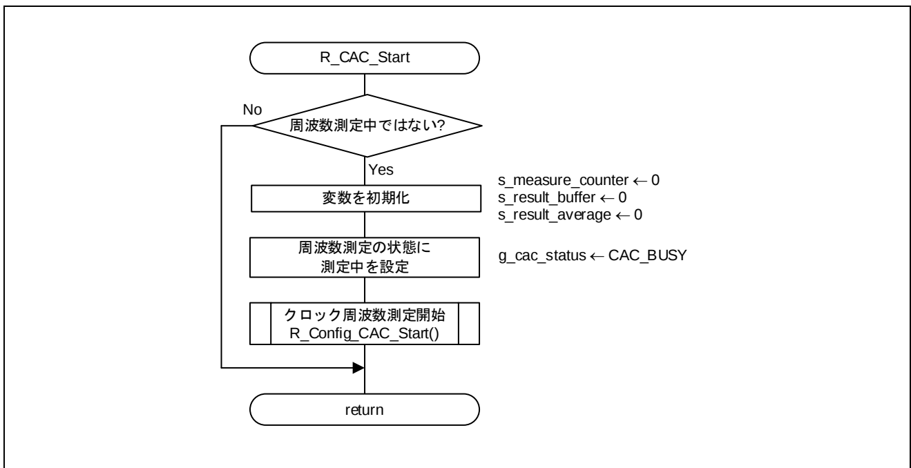
図 4.4 CAC の測定開始処理
