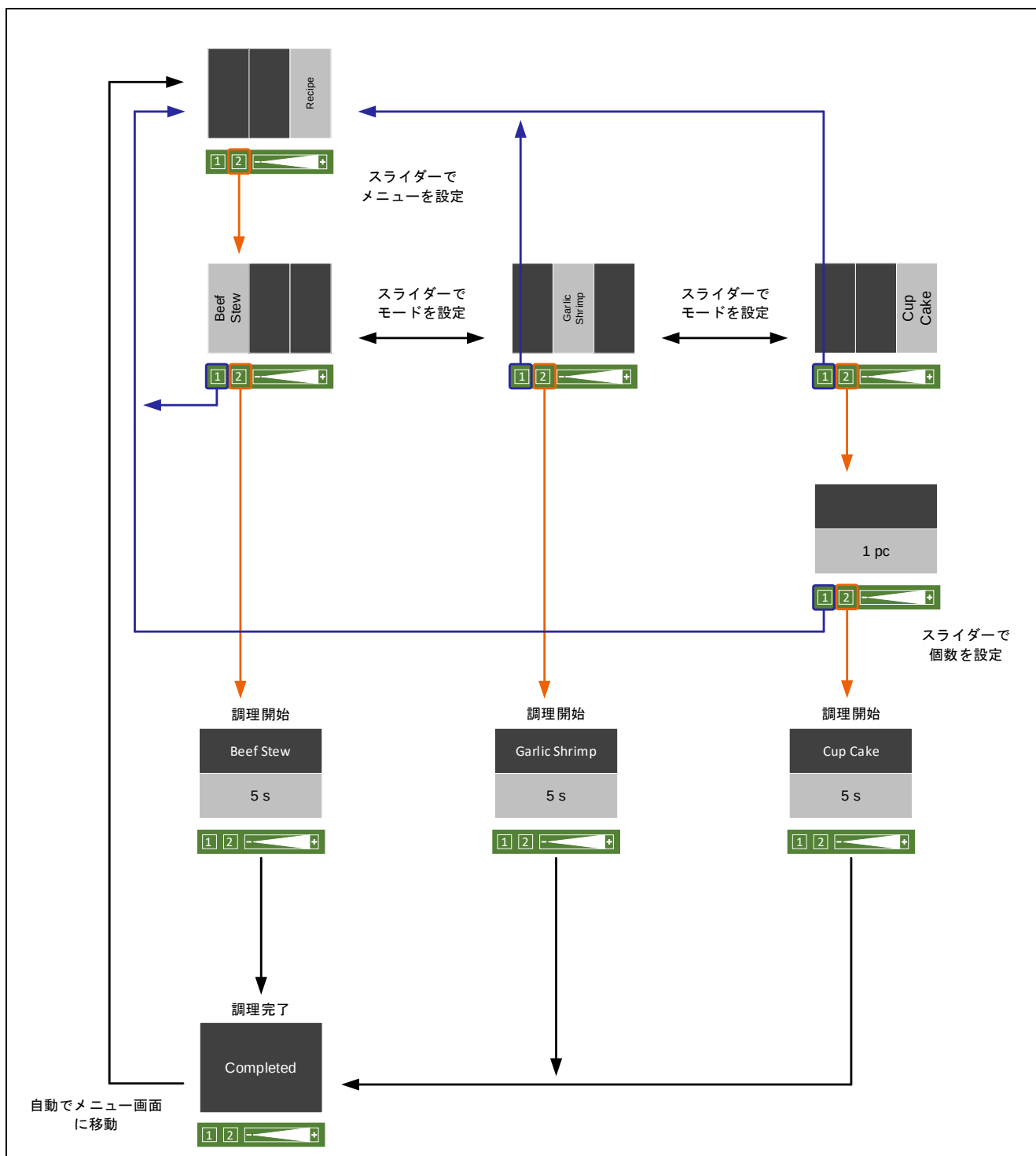
図 4-3 デモ画面のフローチャート (Recipe)
