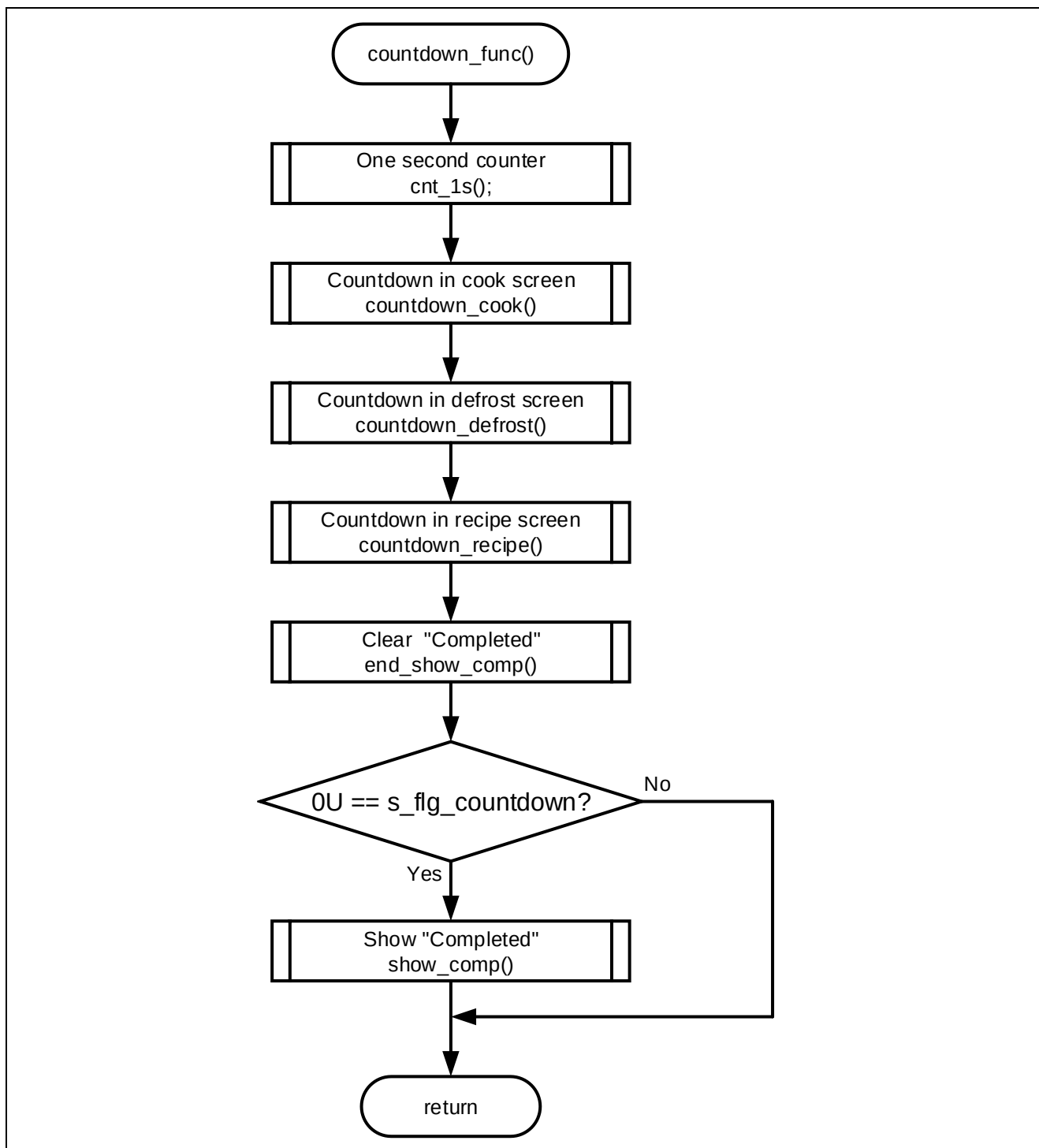
図 4-12 調理中のフローチャート
