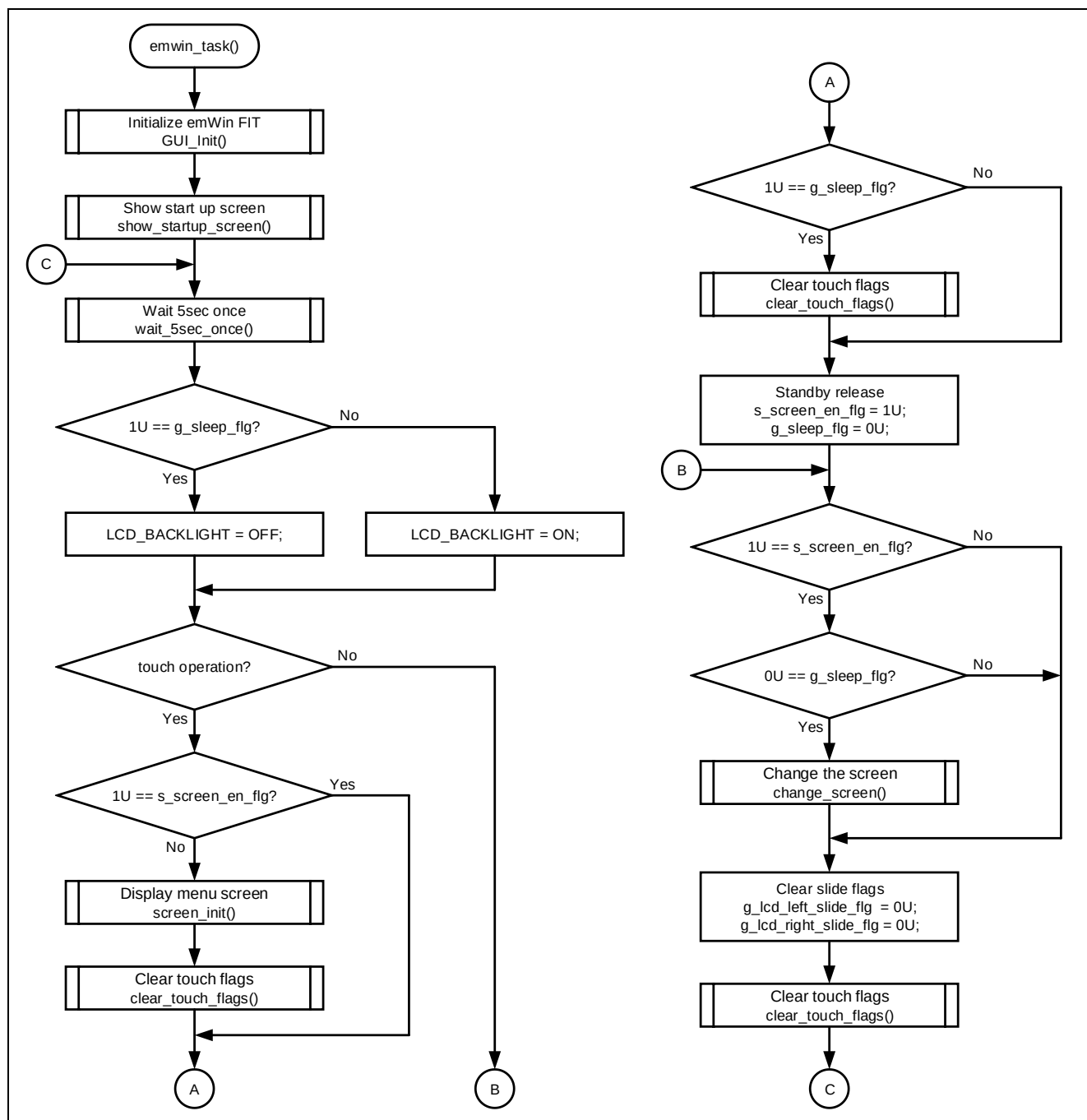
図 4-4 LCD 制御のフローチャート
