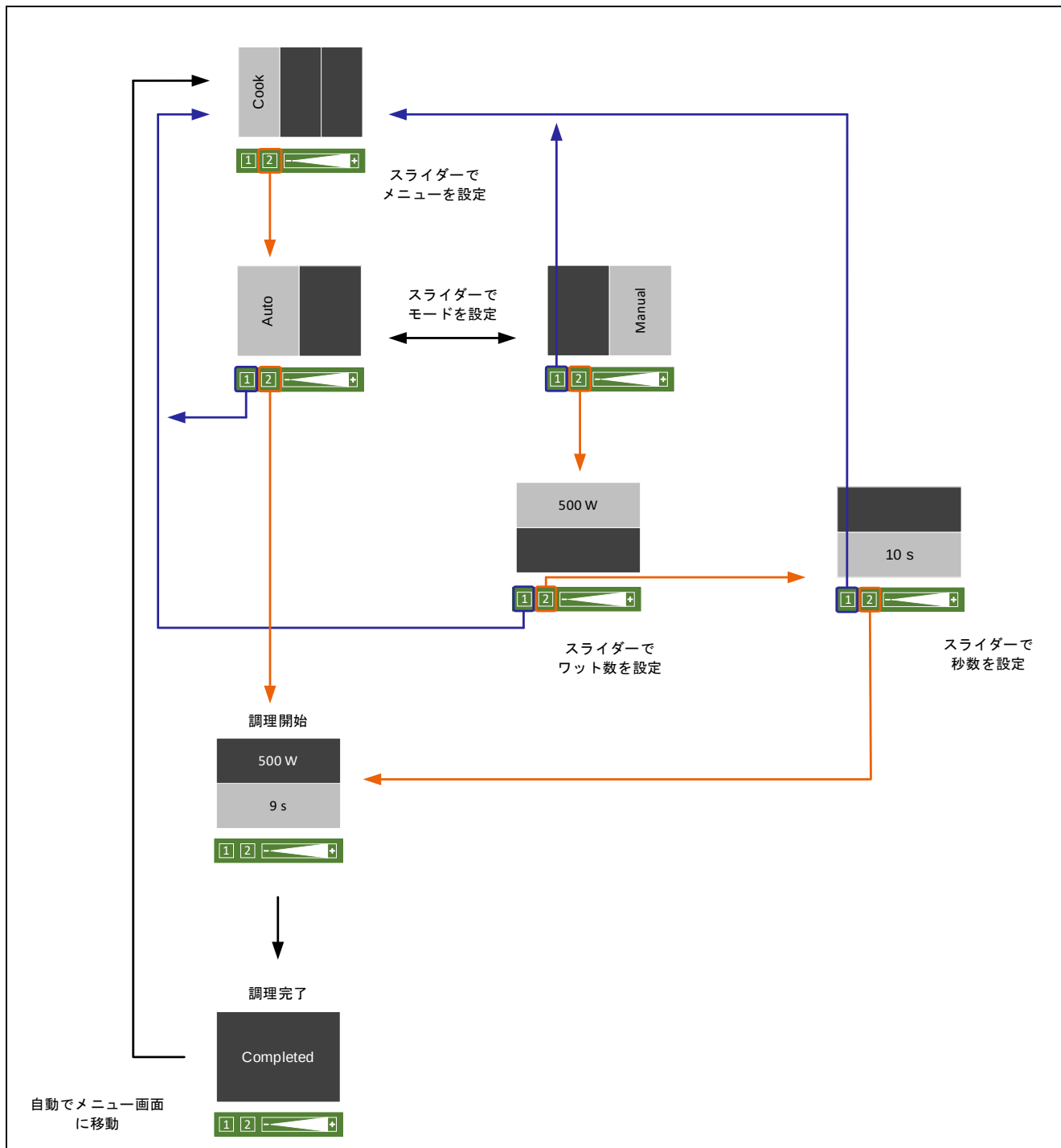
図 4-1 デモ画面のフローチャート (Cook)
