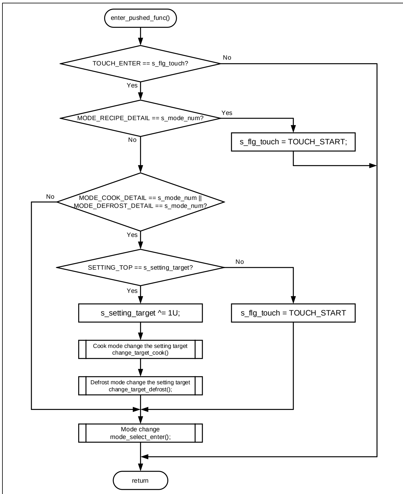
図 4-10 「2」 ボタンタッチ時のフローチャート
