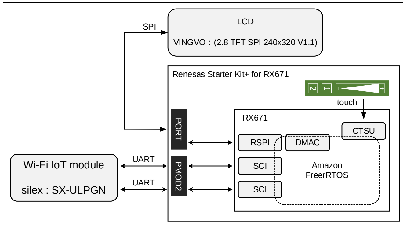
図 1-1 システムの構成
