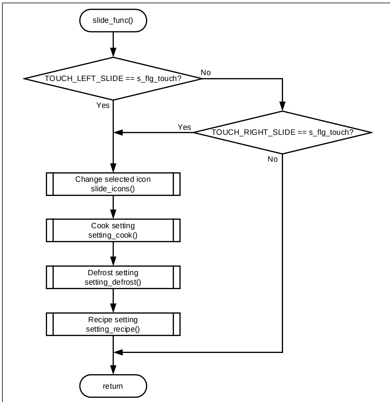
図 4-8 タッチスライダー操作時のフローチャート
