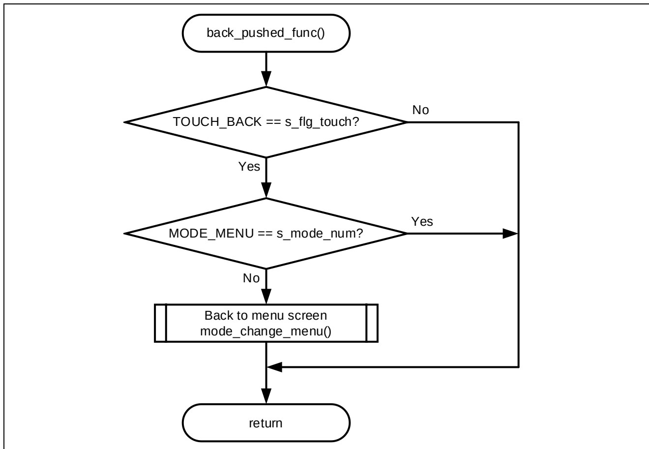
図 4-9 「1」 ボタンタッチ時のフローチャート
