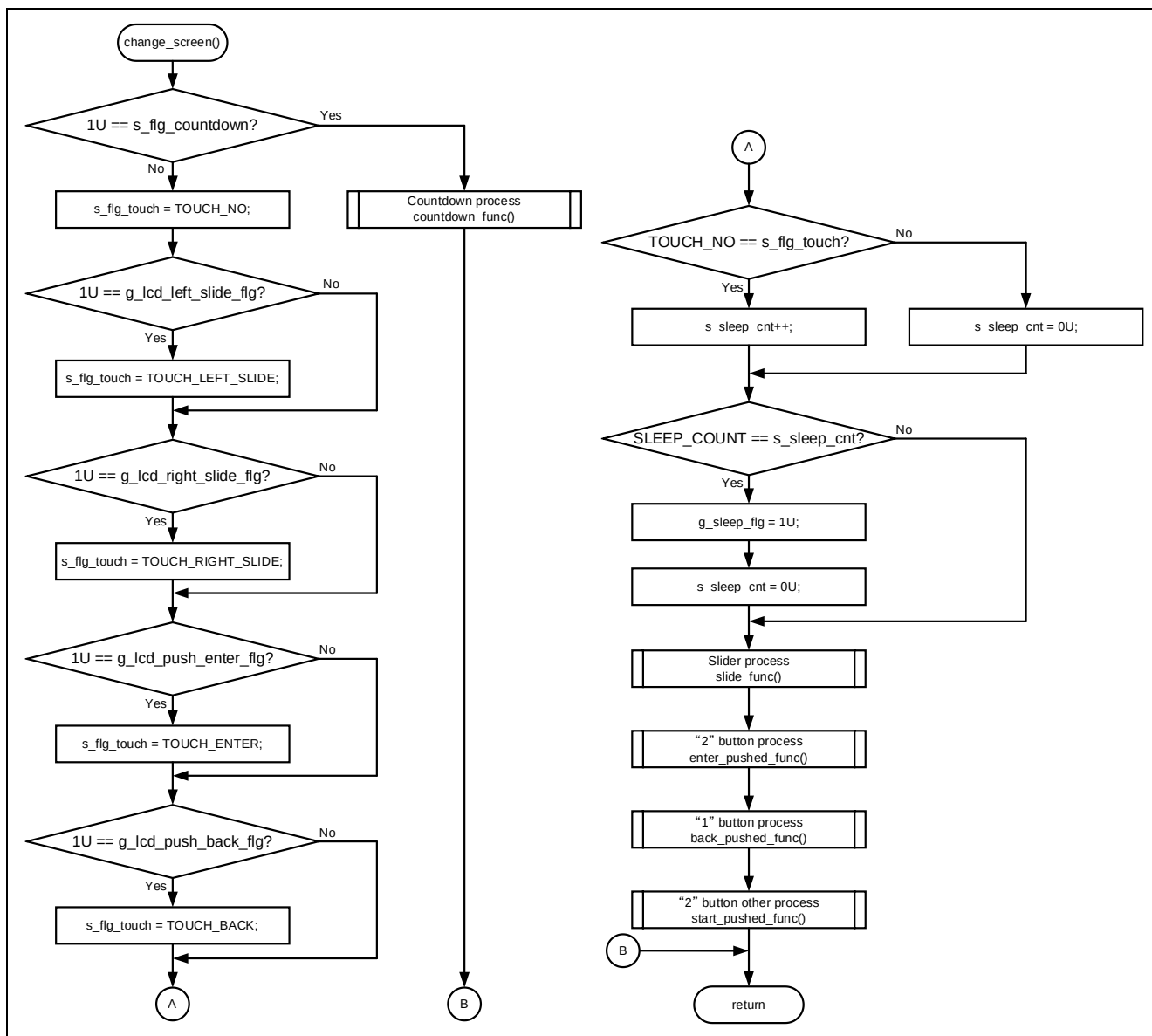
図 4-7 タッチ操作時の処理のフローチャート
