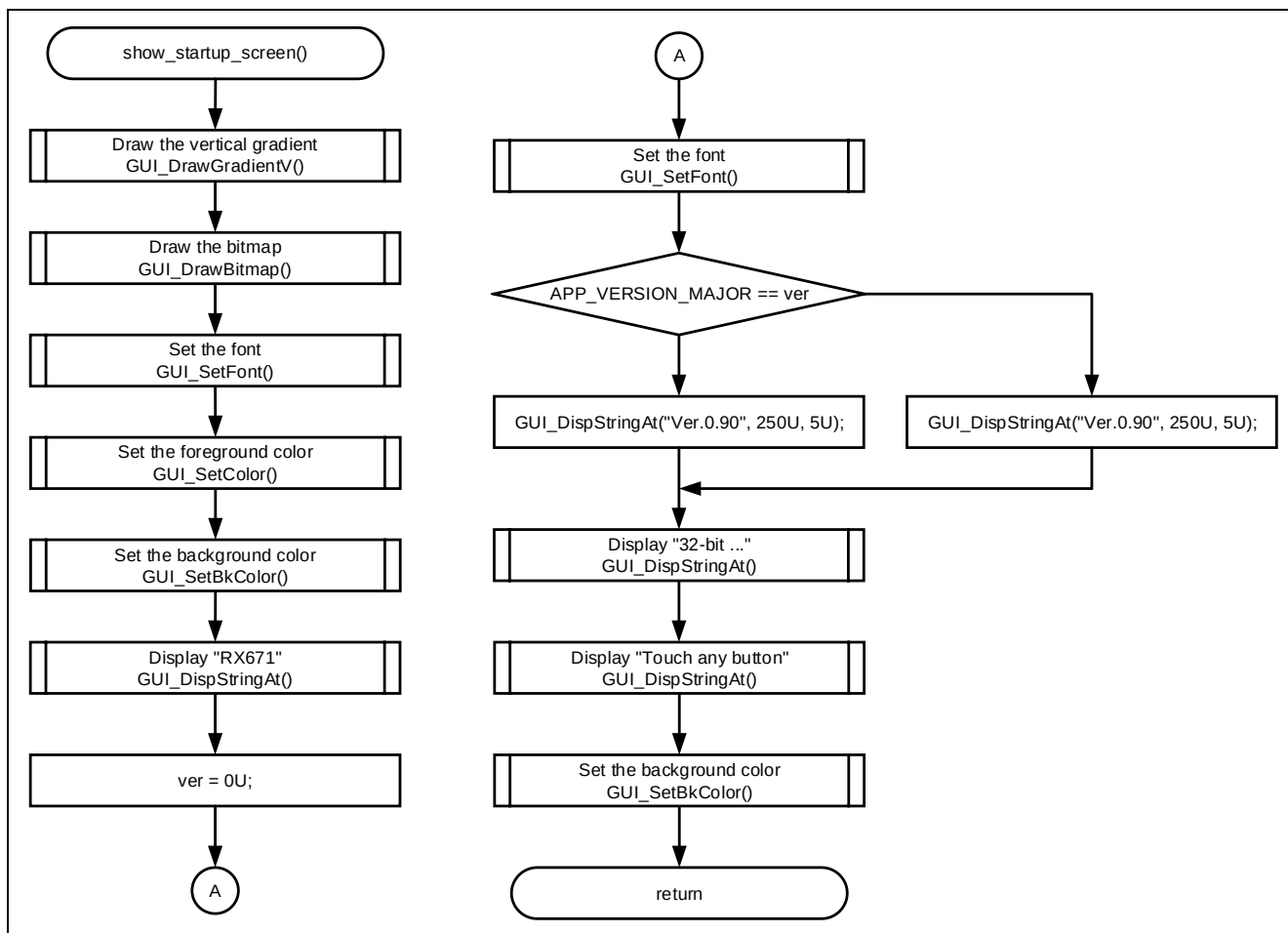
図 4-15 初期画面表示のフローチャート
