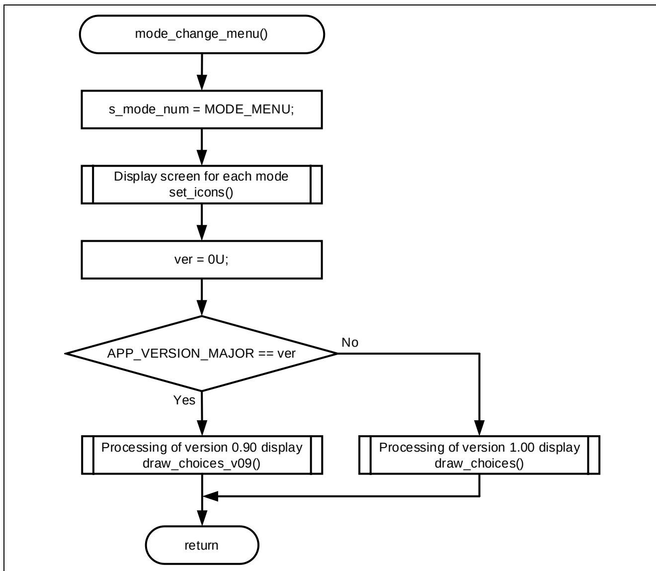
図 4-6 メニュー画面移動時のフローチャート
