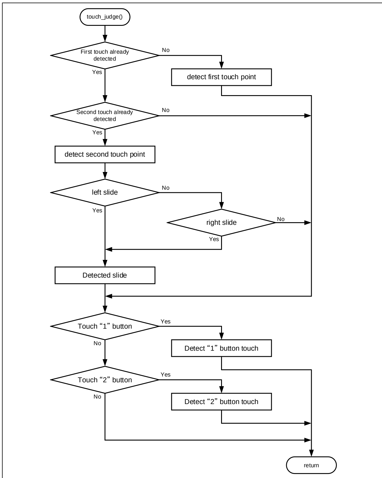
図 4-14 タッチ判定のフローチャート
