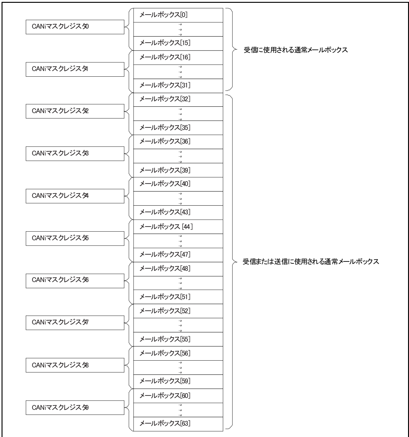
図 19. 通常メールボックスモードのメールボックス構造
