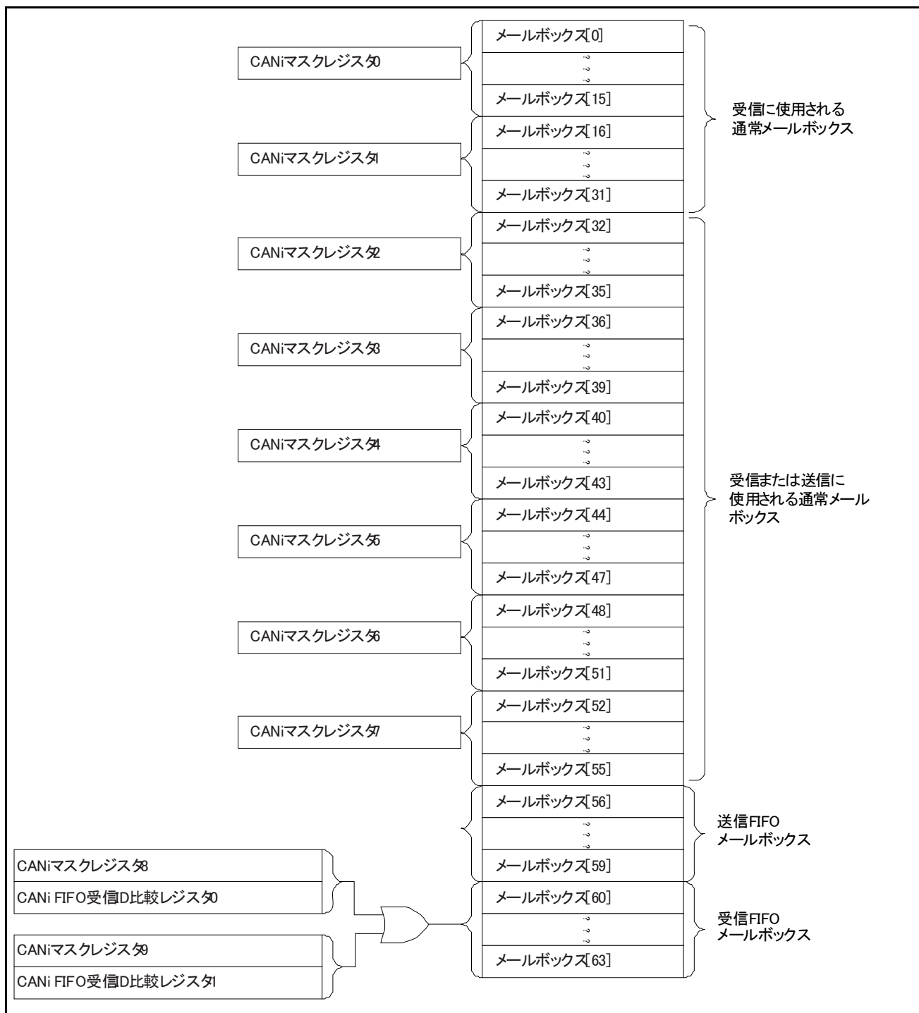
図 20. FIFO メールボックスモードのメールボックス構造
