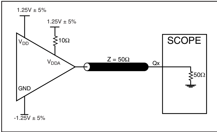
2.5V LVCMOS/LVTTL Output Load AC Test Circuit
