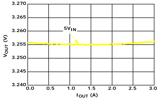
図 10. 負荷レギュレーション、 V_{OUT} = 3.3\text{V} 、 T_A = +25^\circ\text{C}
