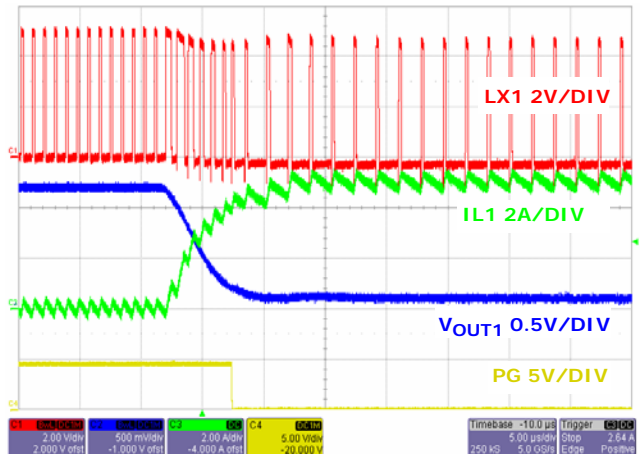
図 28. 出力短絡、チャンネル 1
