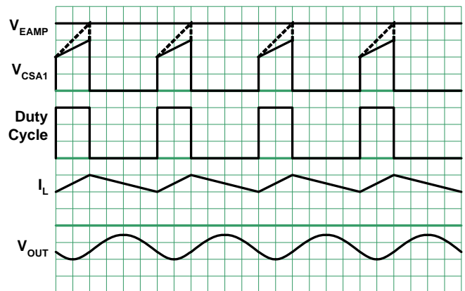
図 40. PWM 動作波形
