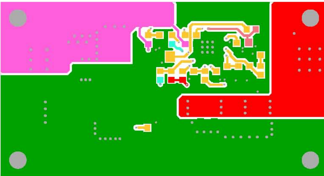
FIGURE 27. BOTTOM LAYER
