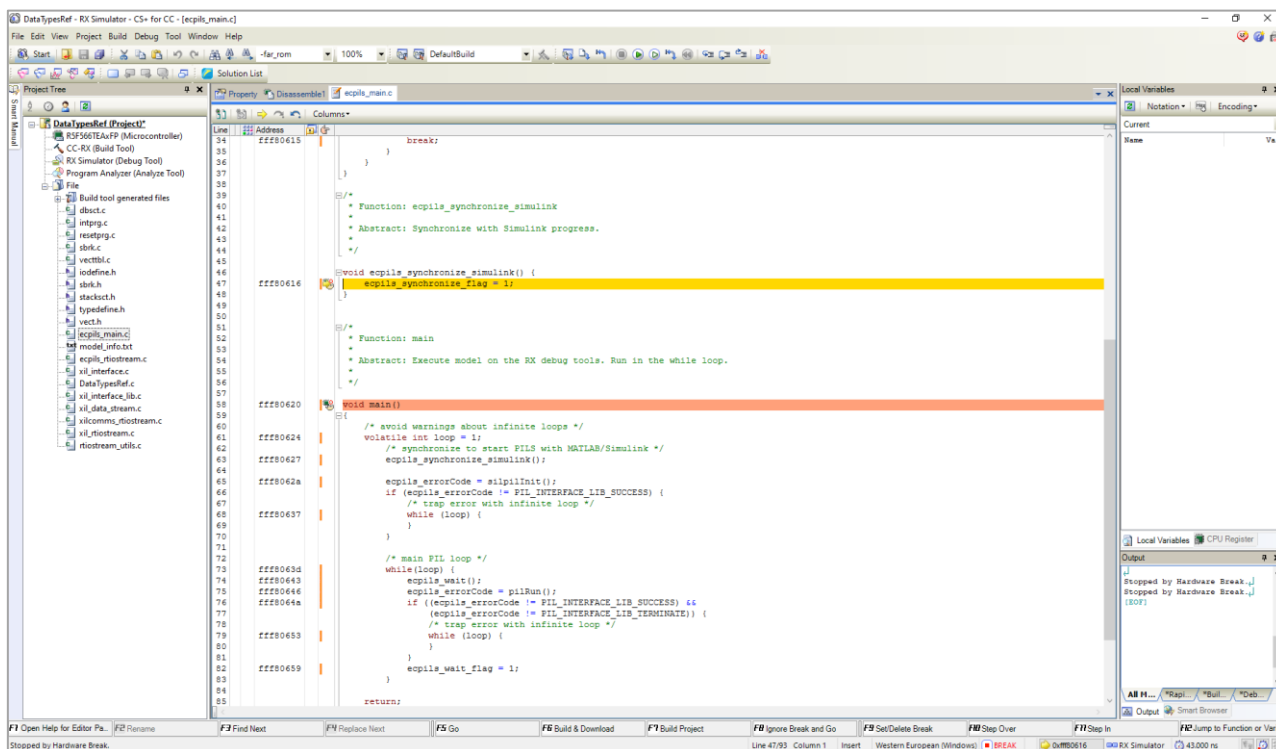
図 3-28 ecplis_main.cに自動的に設定される2つのブレーク・ポイント(CS+)
