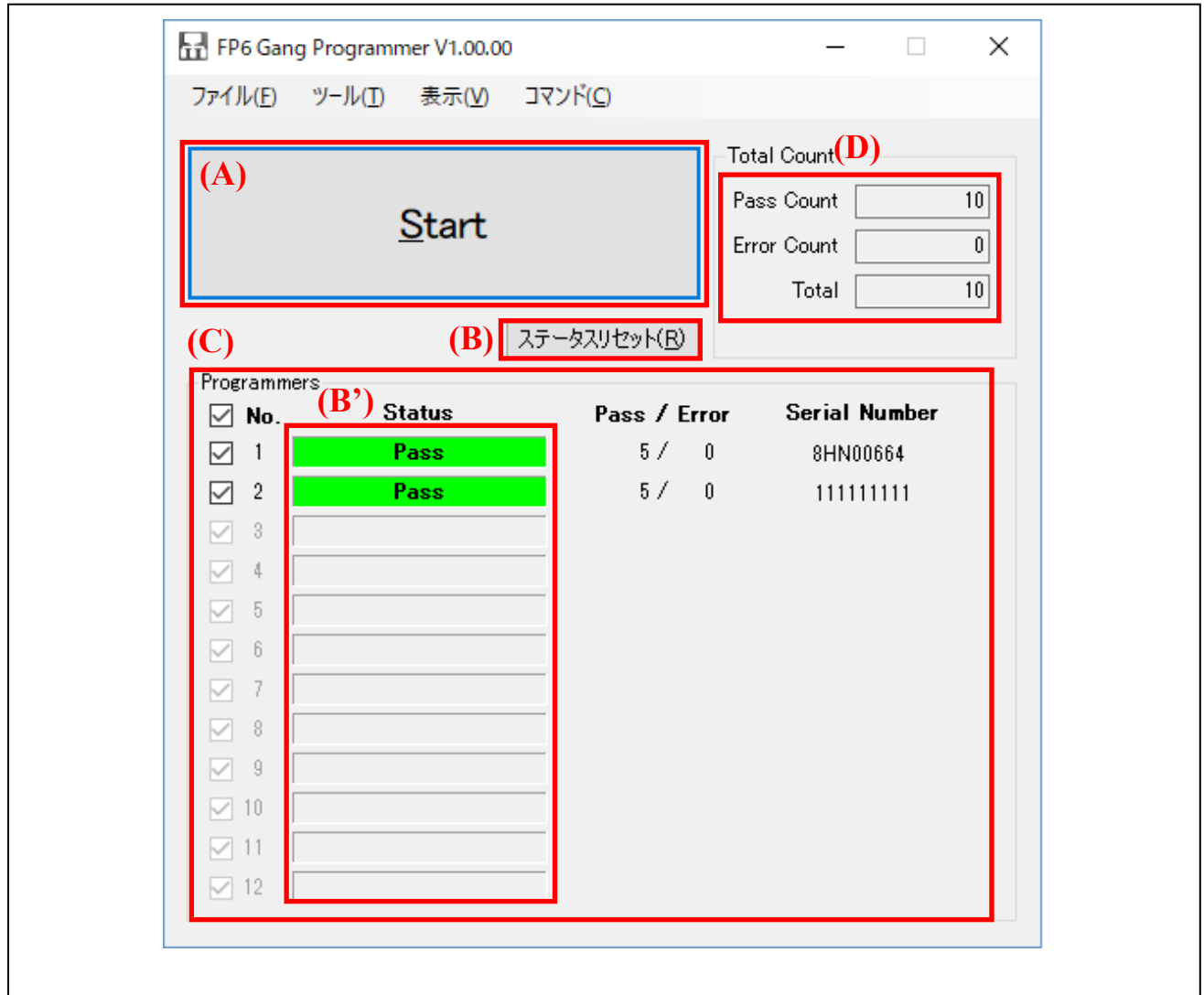
図 5 メインウィンドウ
