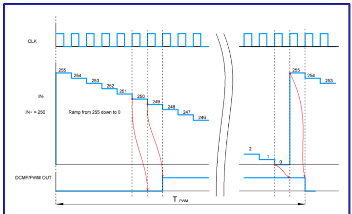
PWM モードの DCMP/PWM
