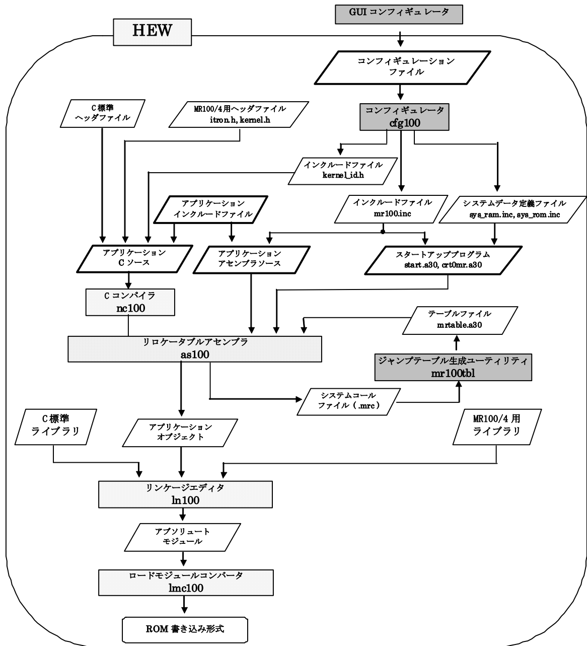
図 6.1 MR100 システム生成フロー
