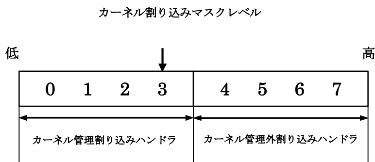
図 3.22 割り込みハンドラの IPL
