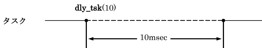
図 4.9 dly_tsk サービスコール
