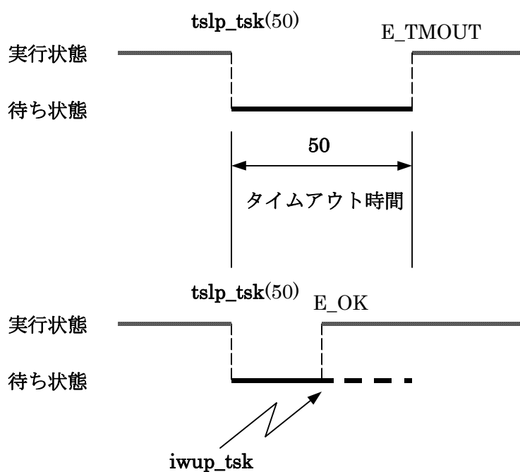
図 4.25 タイムアウト処理
