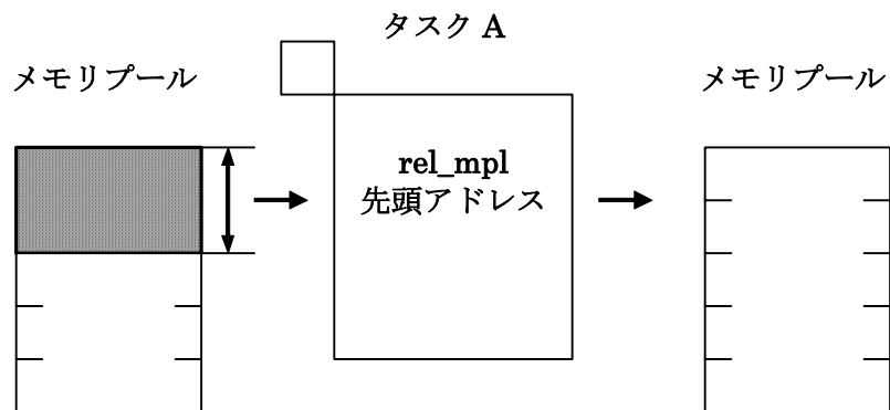
図 4.24 rel_mpl 処理
