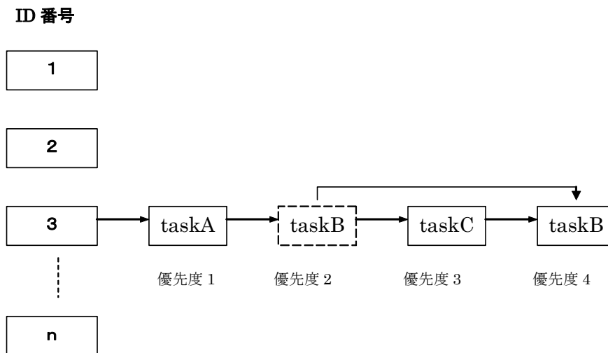
タスク B の優先度を 2 から 4 に変更した場合
