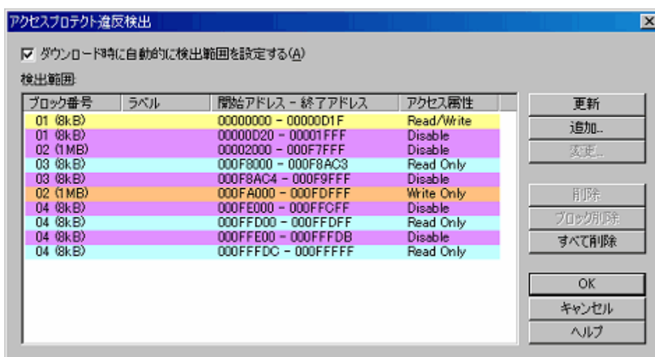
図5.141 [アクセスプロテクト違反検出] ダイアログボックス
