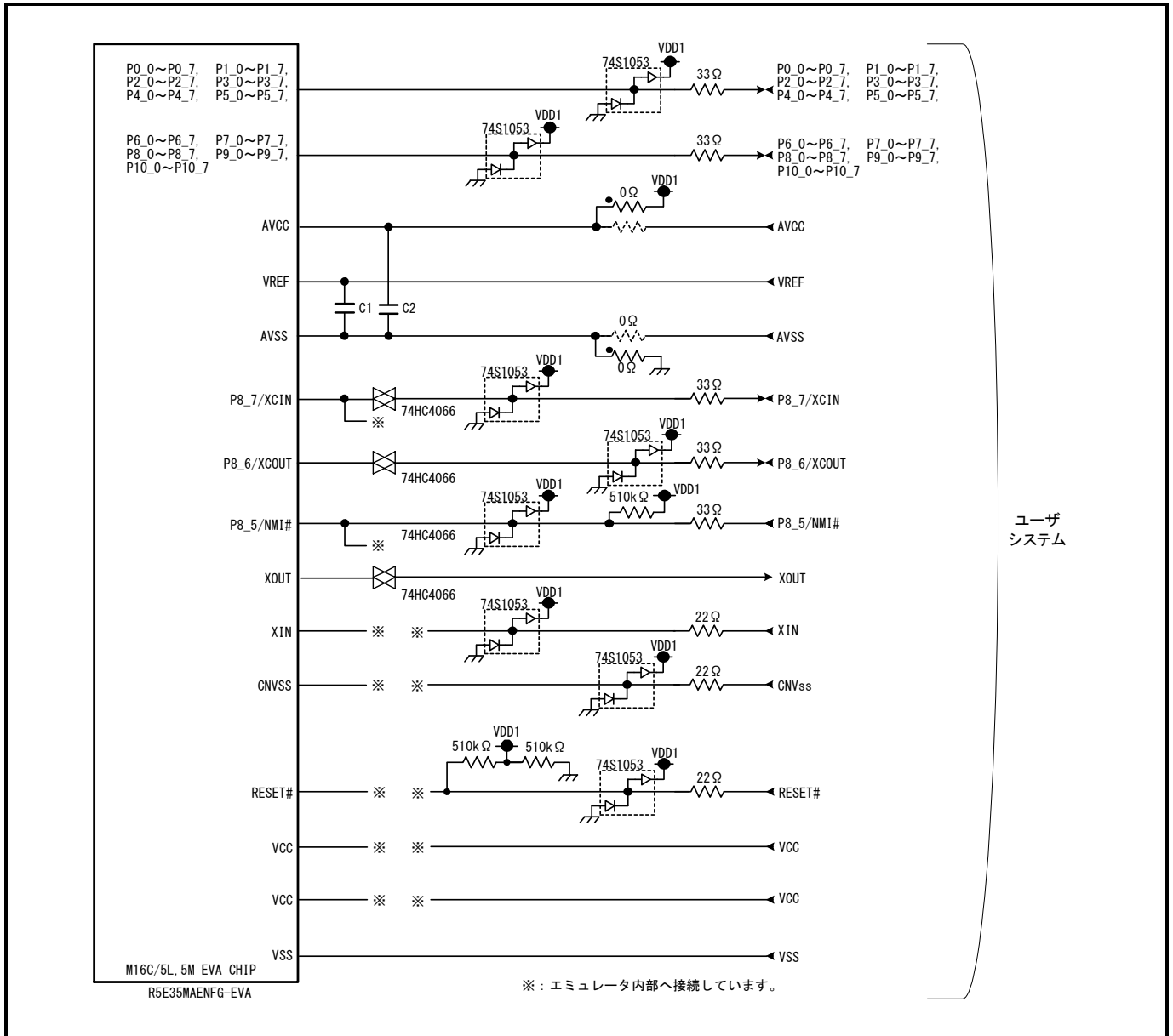
図7.1 ROE535M00MCU00の接続図(一部)
