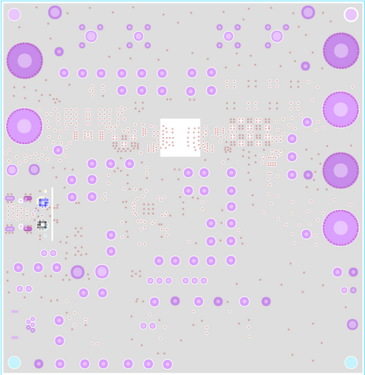
Figure 21. Layer 4
