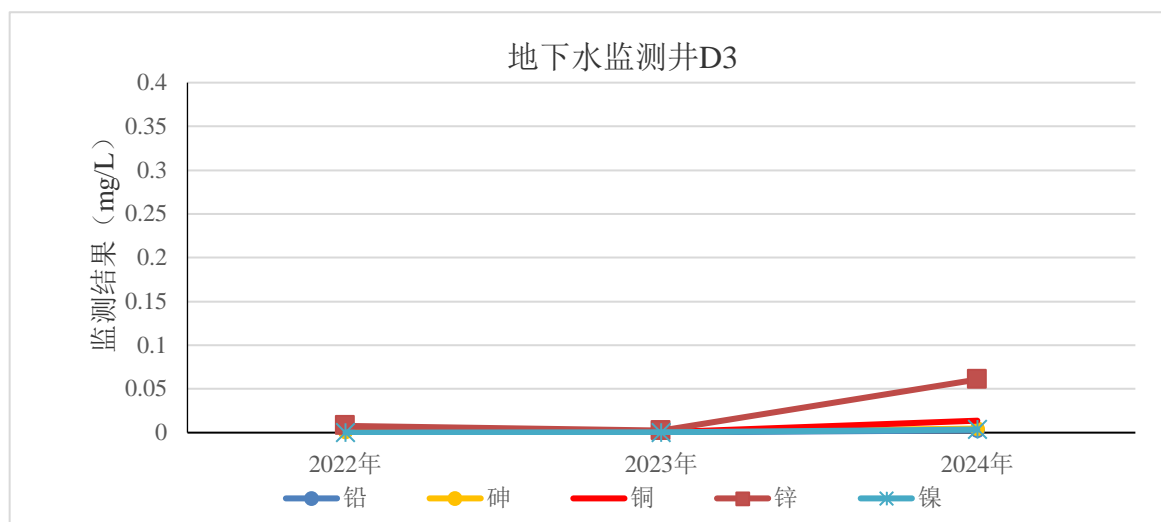
图 8-3 地下水监测井 D3 历年监测结果趋势变化图
