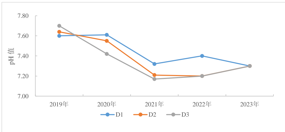
图 2-4 地下水各监测点位 pH 变化趋势图
