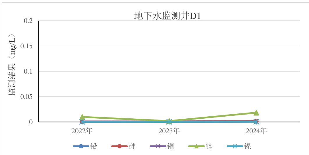
图 8-1 地下水监测井 D1 历年监测结果趋势变化图
