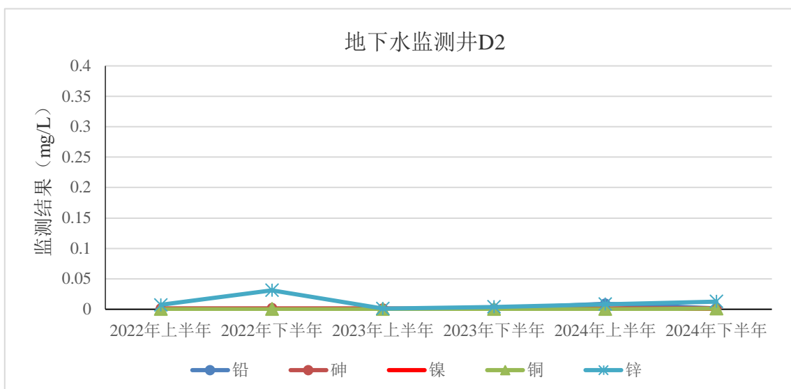
图 8-2 地下水监测井 D2 历年监测结果趋势变化图
