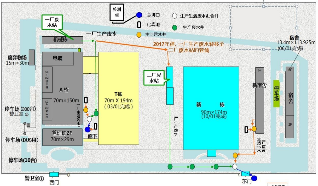
图 4-4 污水管线图
