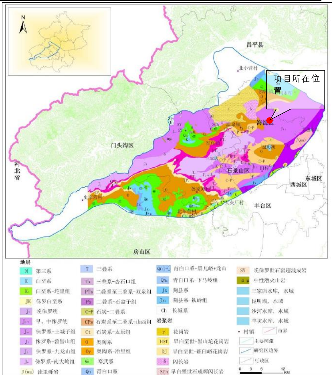
图 6 项目所在区域基岩地质图
