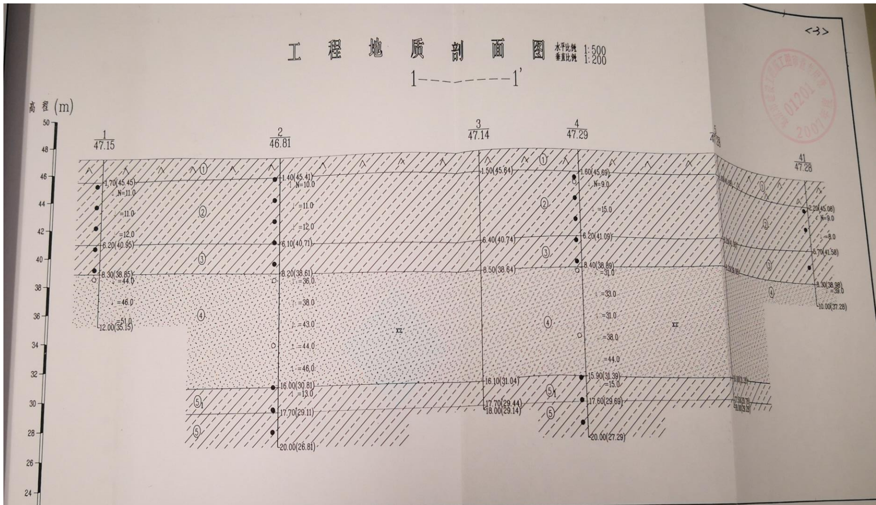
图 8 工程地质剖面图
