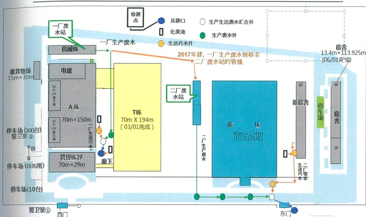
图 4-4 污水管线图
