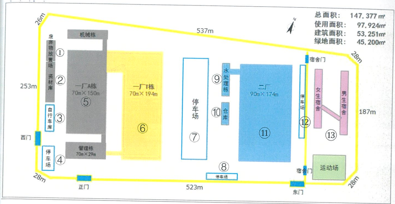
图 10 厂区区域识别
