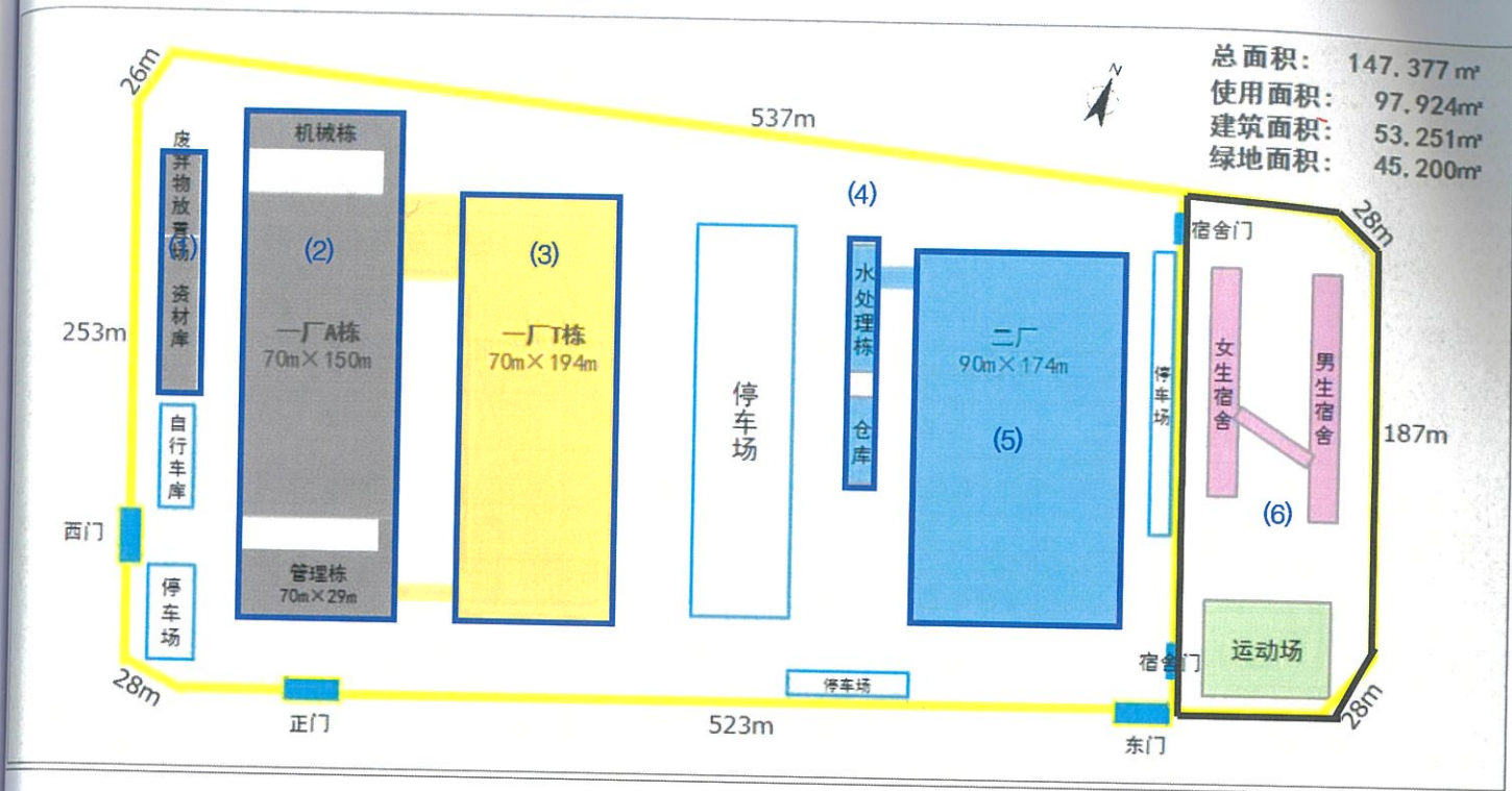
图 11 厂区区域划分
