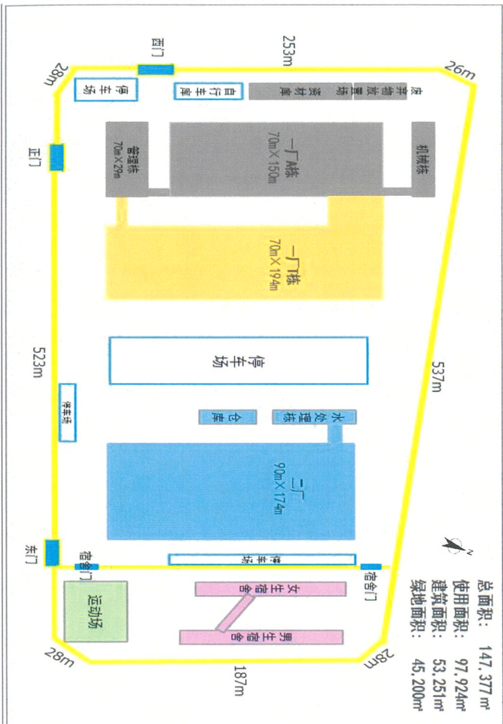
图 2 厂区平面布置图
