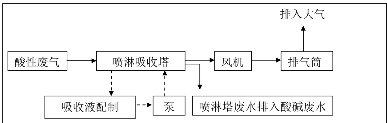
图 2 废气处理工艺流程图
