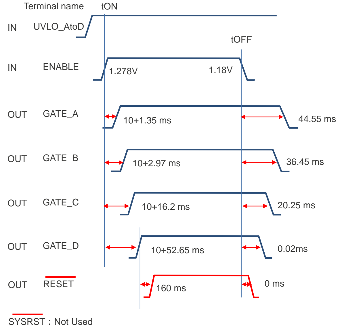
【 Timing chart 】
