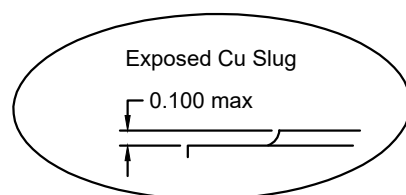
Detail B Scale: 2X
