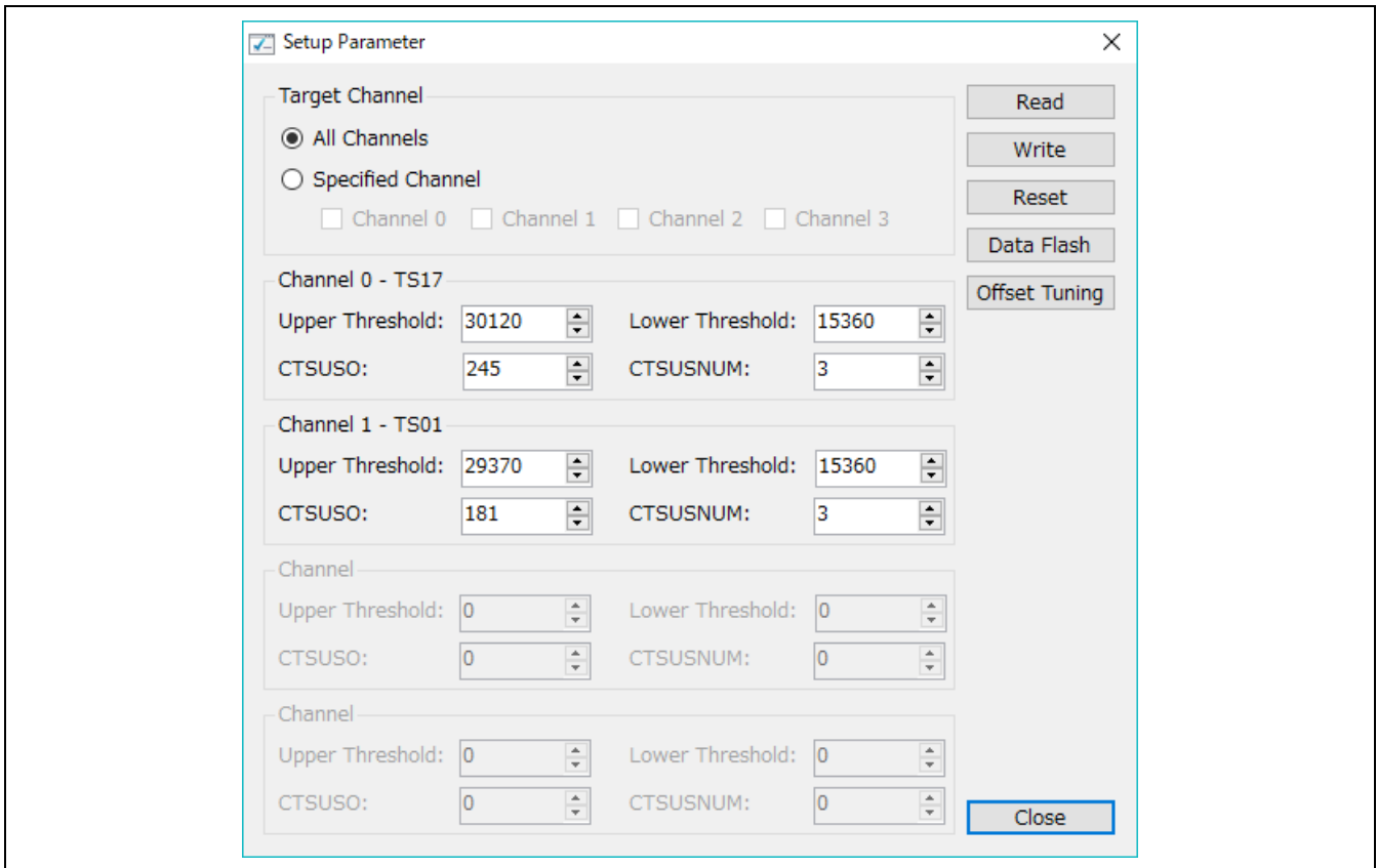
Figure 3.2 Setup Parameter dialog
