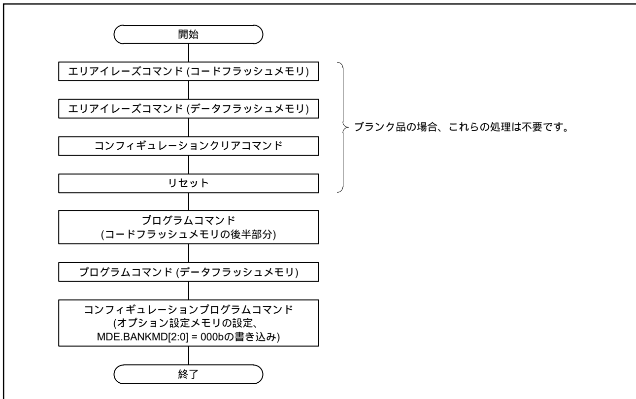
図1 リニアモードのままフラッシュメモリを書き換える例
