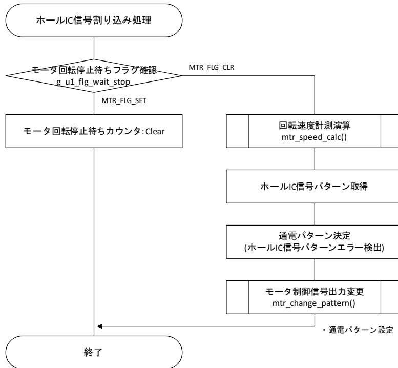
Figure 3-8 フローチャート(ホール IC 信号割り込み処理)
