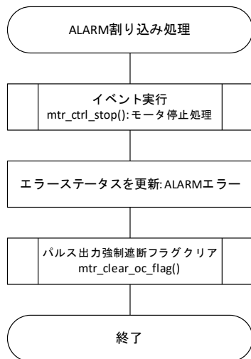
Figure 3-11 フローチャート(ALARM 割り込み処理)
