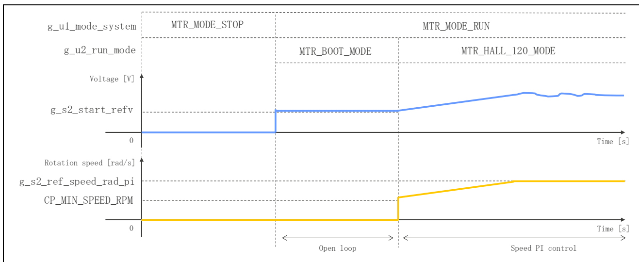
Figure 3-5 始動方法
