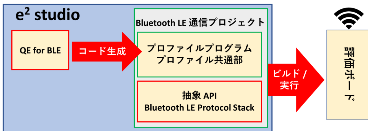
図 1.3 QE for BLE によるプロファイル開発環境 (RX23W, RA4W1 環境)
