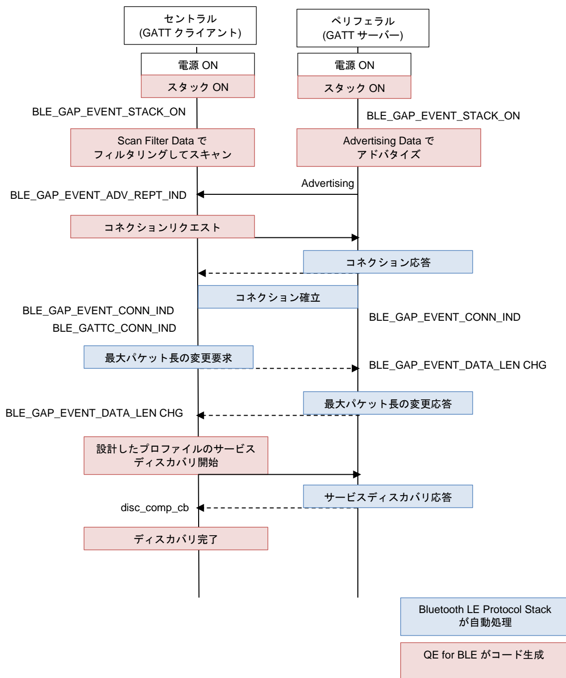
図 4.15 app_main.c に実装されているプログラムの動作
