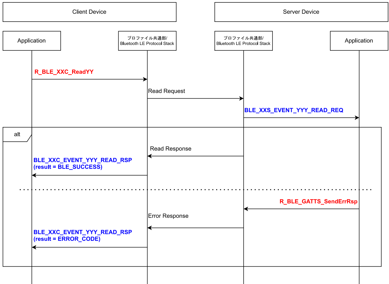
図 4.33 Read 動作時のシーケンスチャート
