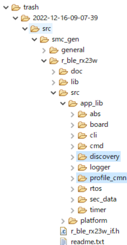
図 6.17 trash フォルダからの復元
