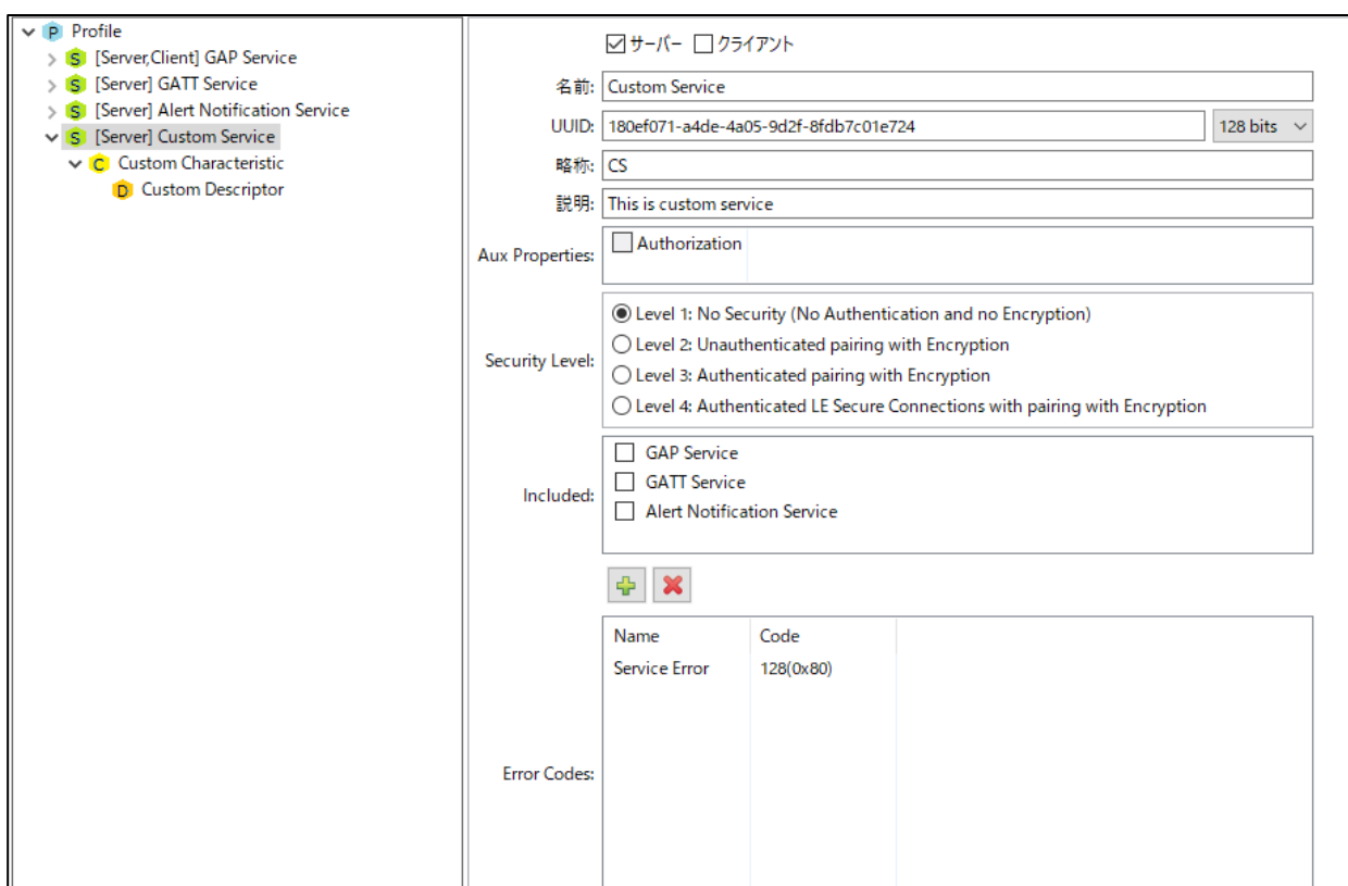
図 3.8 サービスの設定項目
