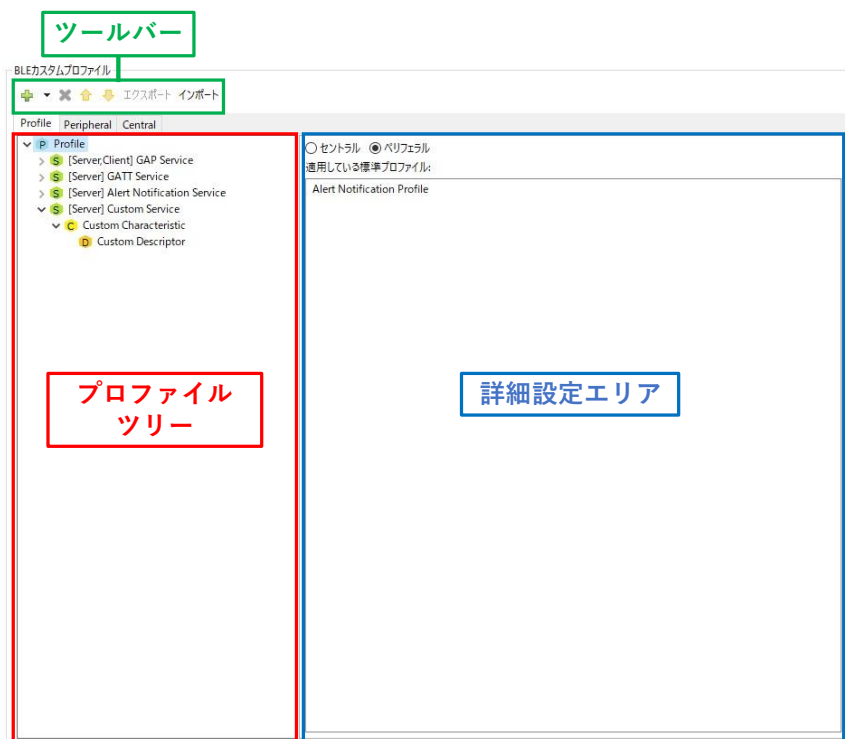
図 3.4 QE for BLE の設定画面
