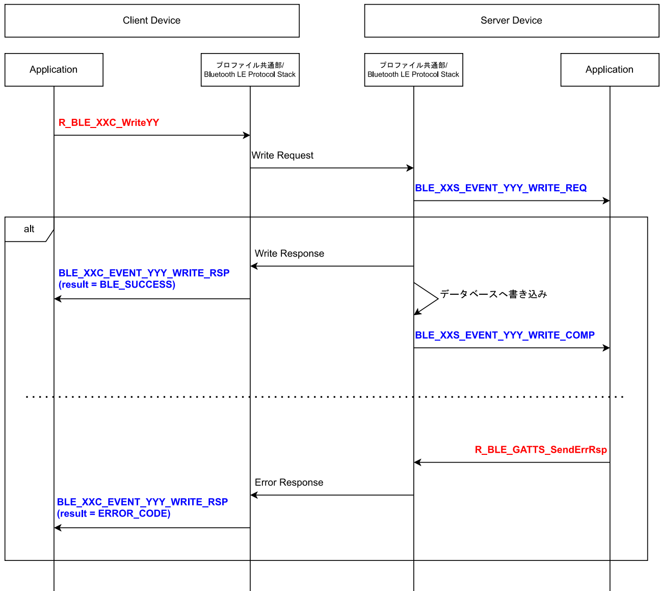
図 4.22 Write 動作時のシーケンスチャート
