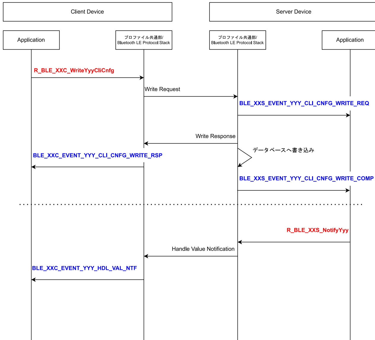
図 4.40 Notify 動作のシーケンスチャート
