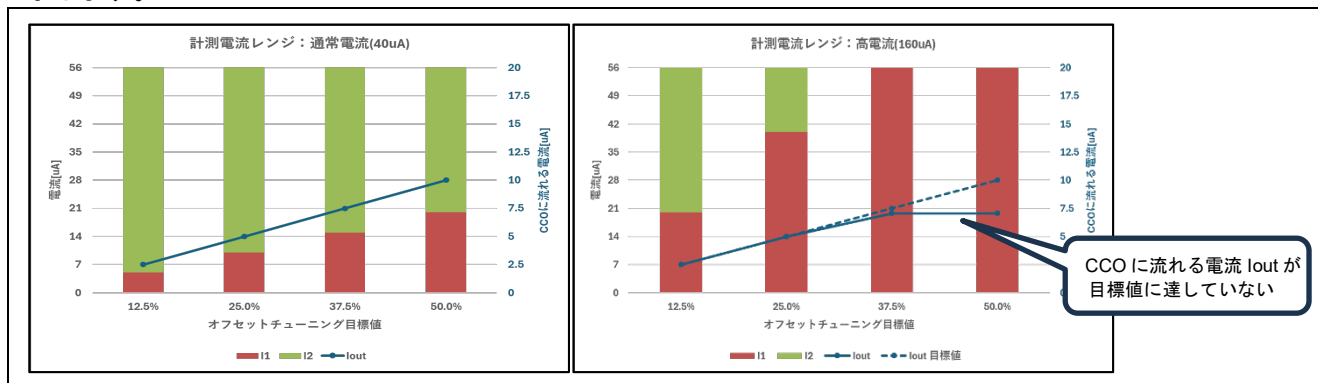
図 3-18 オフセットチューニング目標値と計測電流レンジを変更した際の電流値
