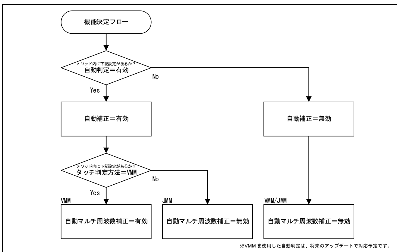
図 3-29 “自動判定/自動補正(ハードウェア)/自動マルチ周波数補正(ハードウェア)”の決定フロー
