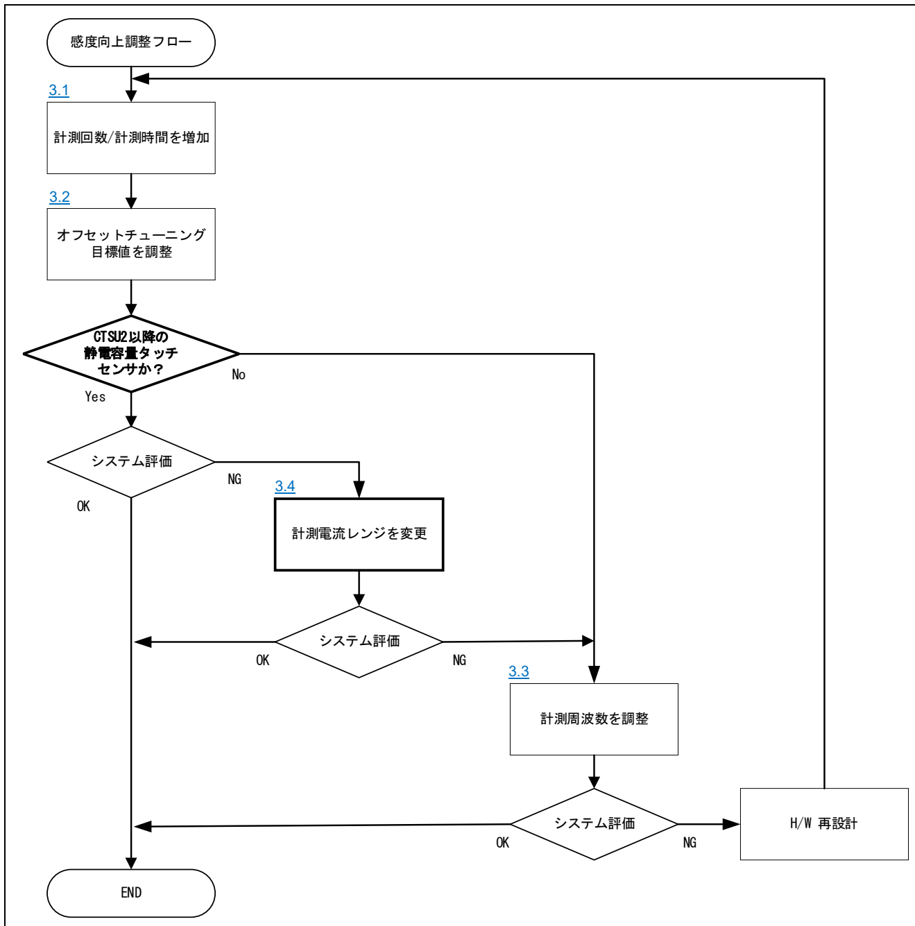
図 2-1 感度向上調整フロー
