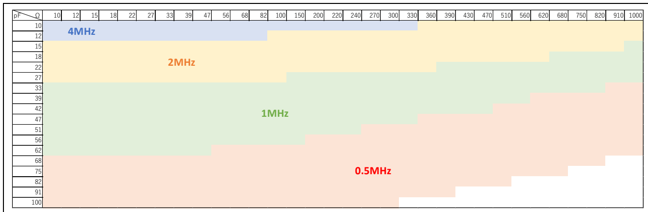
図 3-8 RX130(受信電極 1.6V)の寄生容量/ダンピング抵抗と計測周波数の関係
