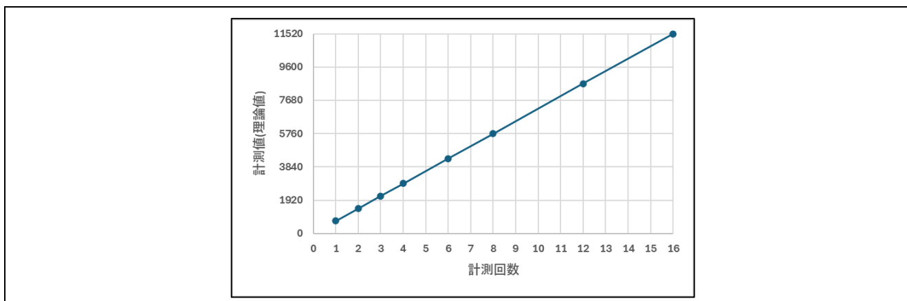
図 3-4 RX140 での“計測回数/計測時間”に対しての計測値(理論値)
