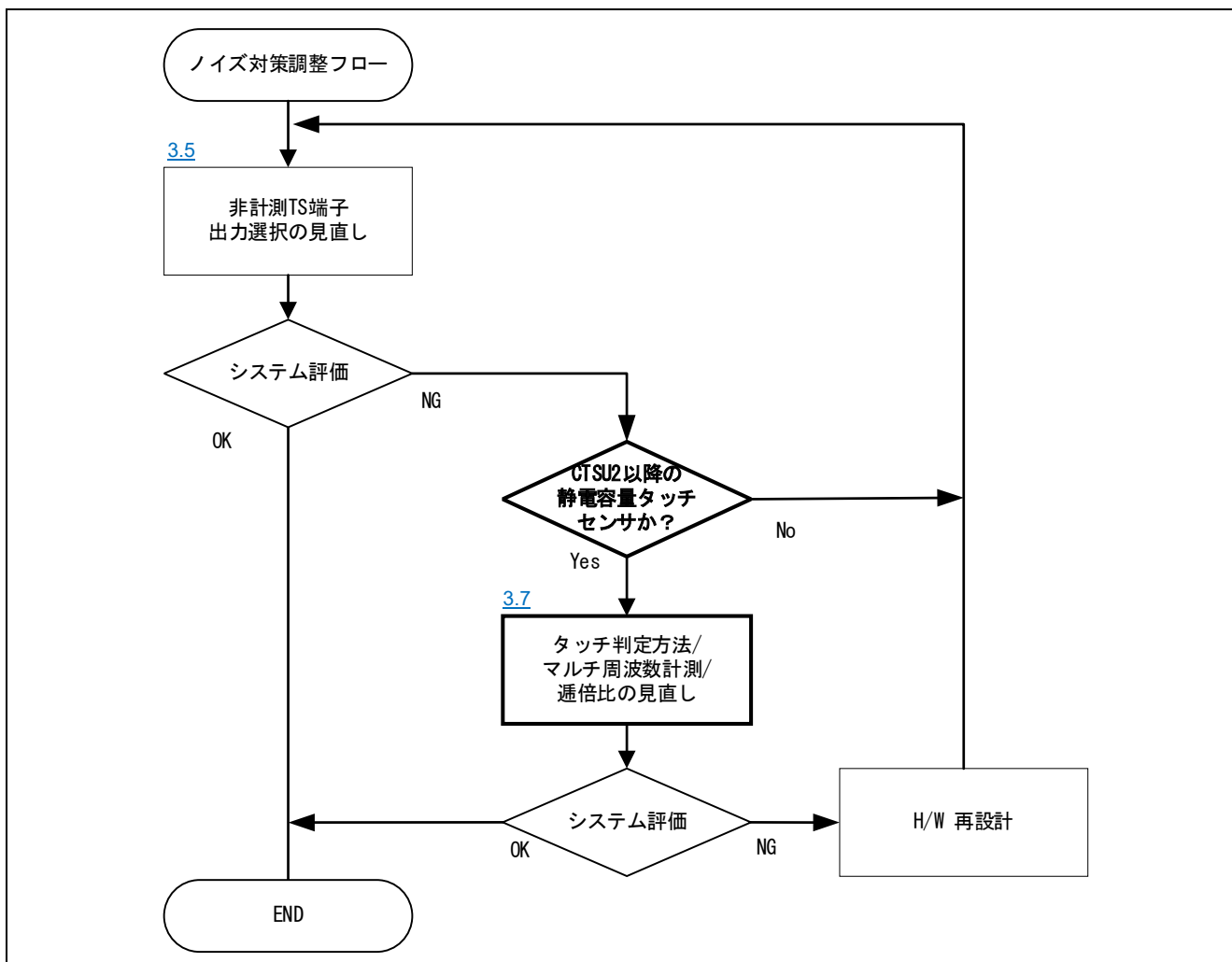
図 2-2 ノイズ対策調整フロー
