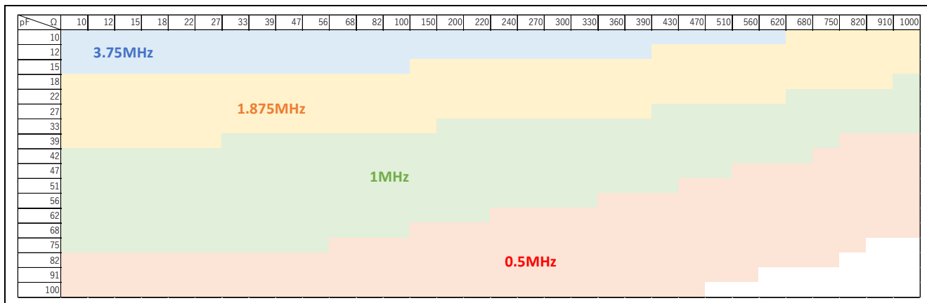
図 3-9 RX671 (受信電極 1.18V)の寄生容量/ダンピング抵抗と計測周波数の関係
