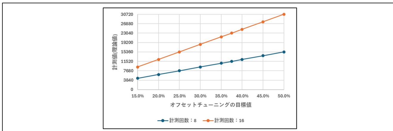
図 3-7 計測回数を変更した場合の“オフセットチューニング時の目標値”に対しての計測値(理論値)
