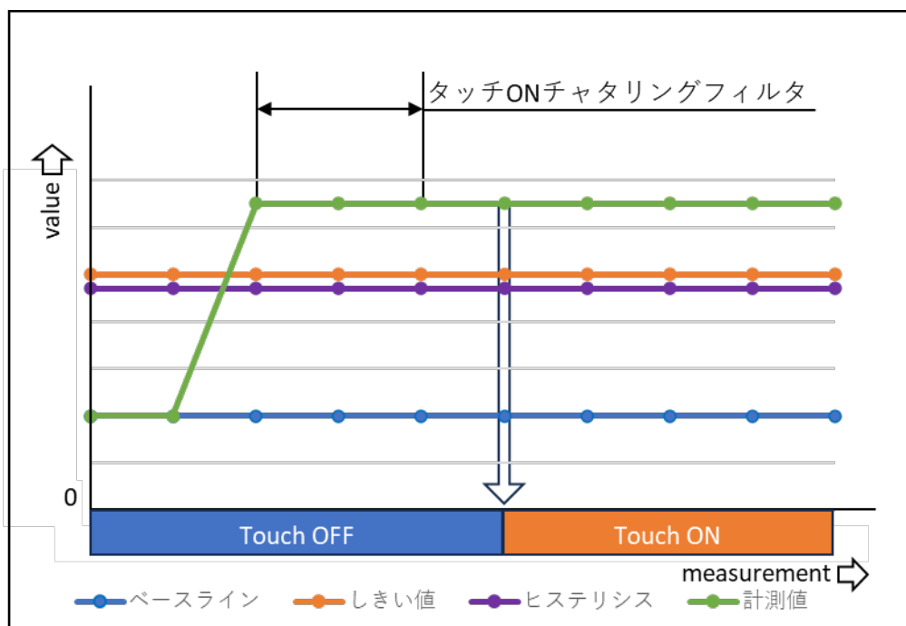
図 3-9 自己容量方式タッチ ON 判定の関係
