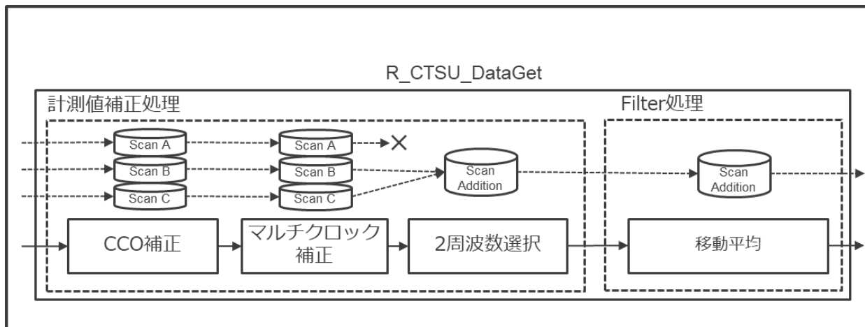
図 3-3 CTSU2 VMM での計測値処理
