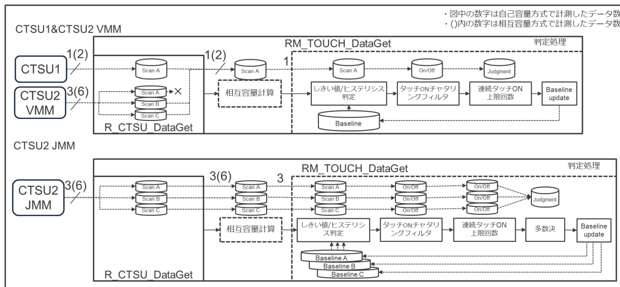
図 3-5 判定処理
