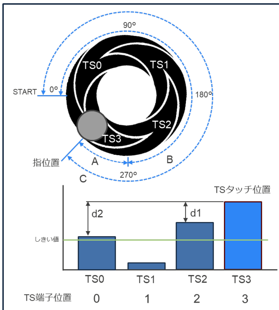
図 3-16 ホイール判定の図
