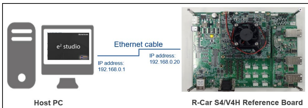
図 2-1 Host PC と Reference Board の接続図
