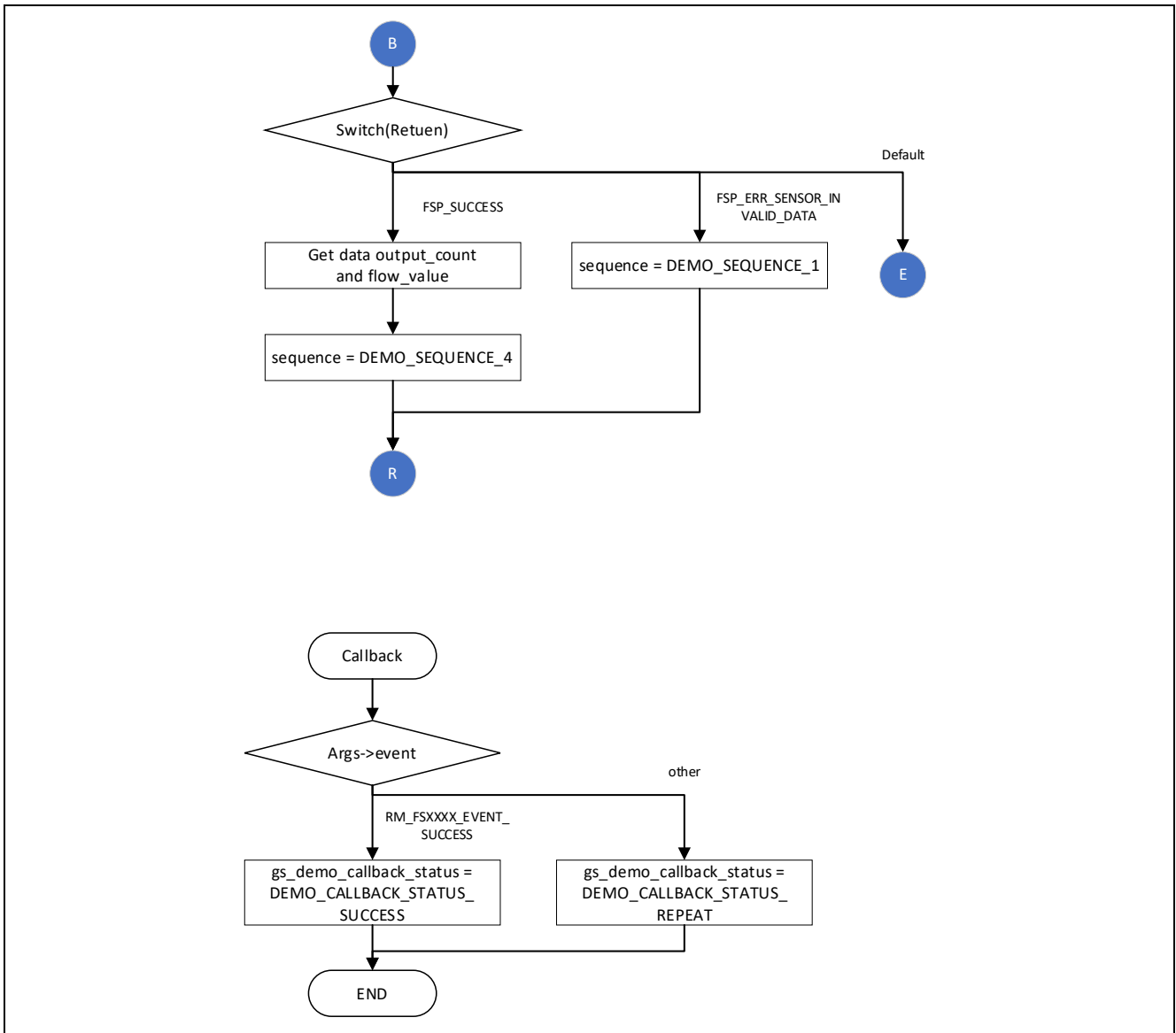
図 4-4 サンプルソフトウェア Non-OS 版メイン処理フロー2
