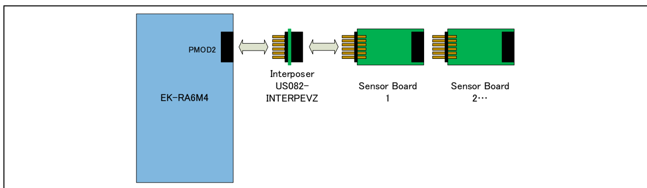
図 2-1 HW 接続図
