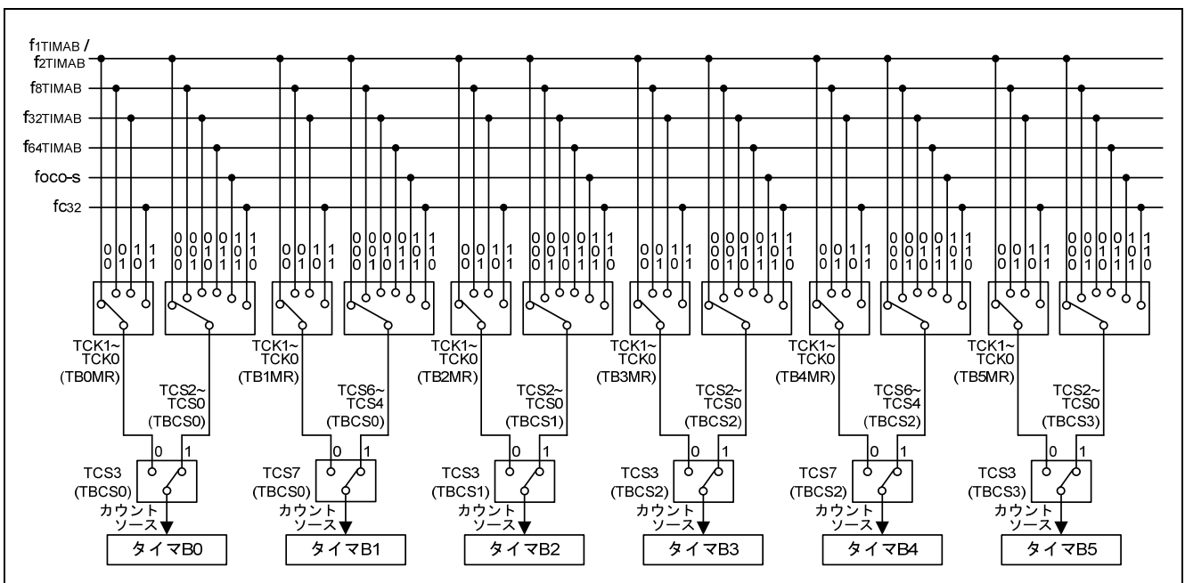
図 2. タイマ B 内部カウントソース
