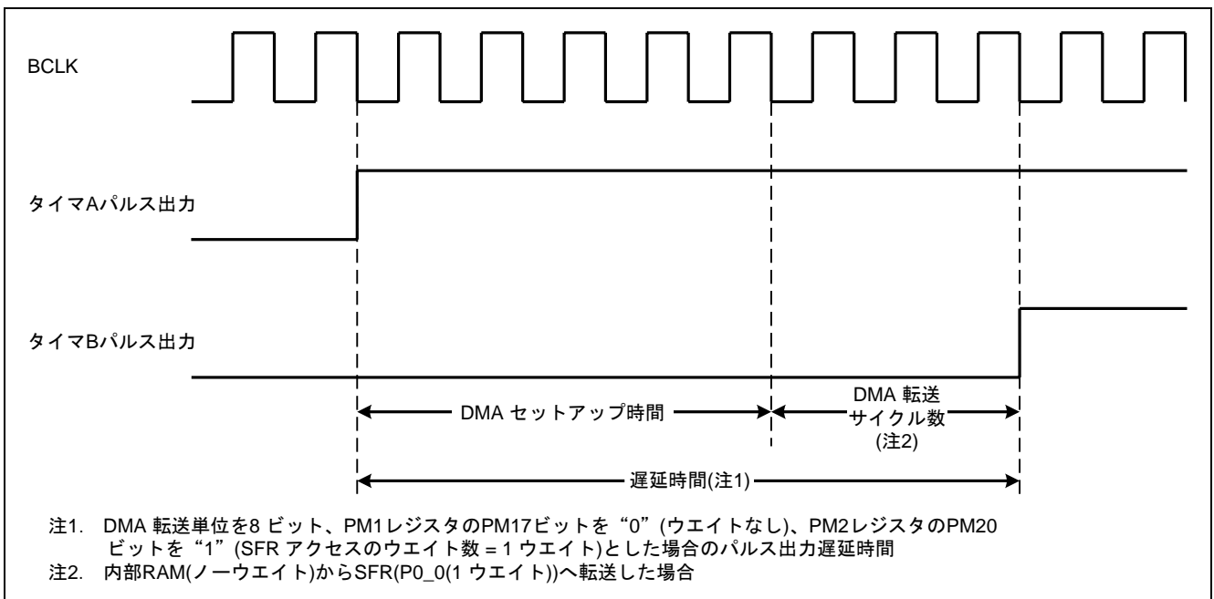
図 3. パルス出力遅延例
