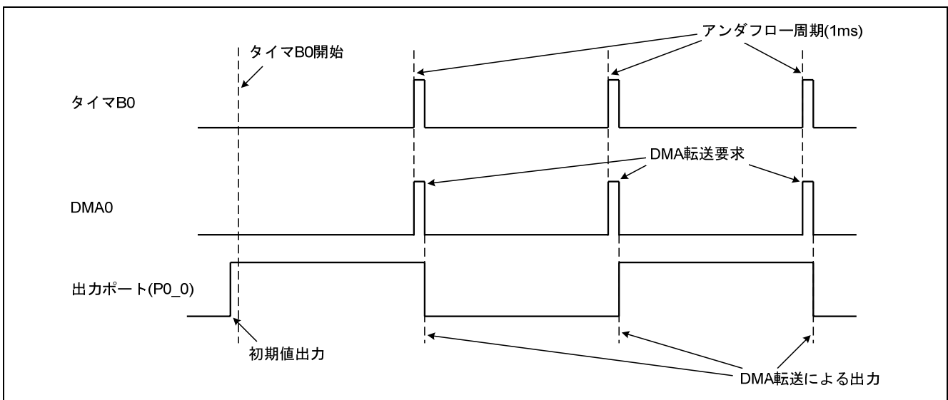
図 1. パルス出力タイミングチャート
