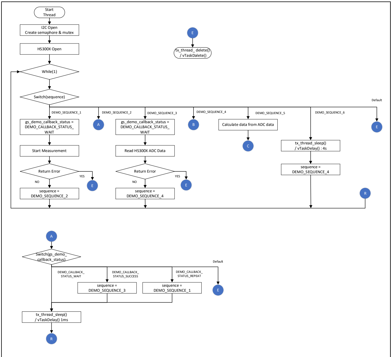
図 4-6 サンプルソフトウェア OS 版メイン処理フロー1
