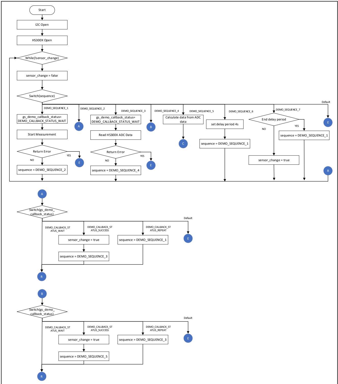
図 4-4 サンプルソフトウェア Non-OS 版メイン処理フロー1
