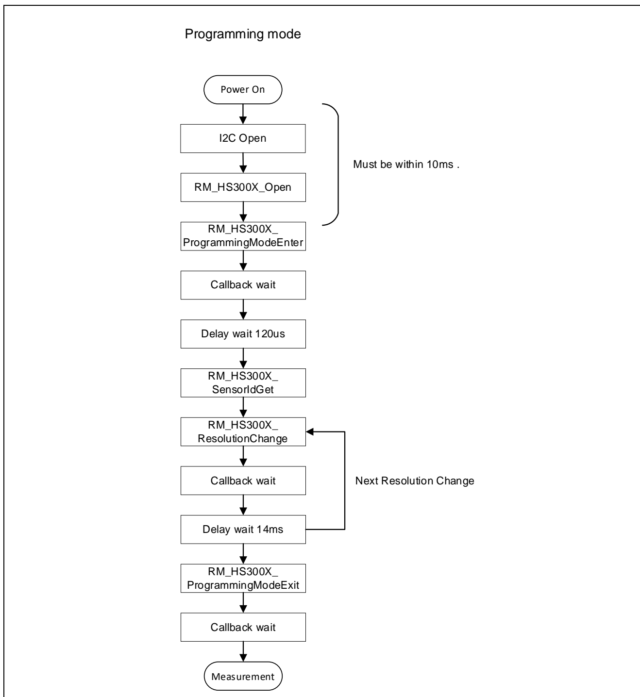
図 4-3 プログラミングモード遷移図
