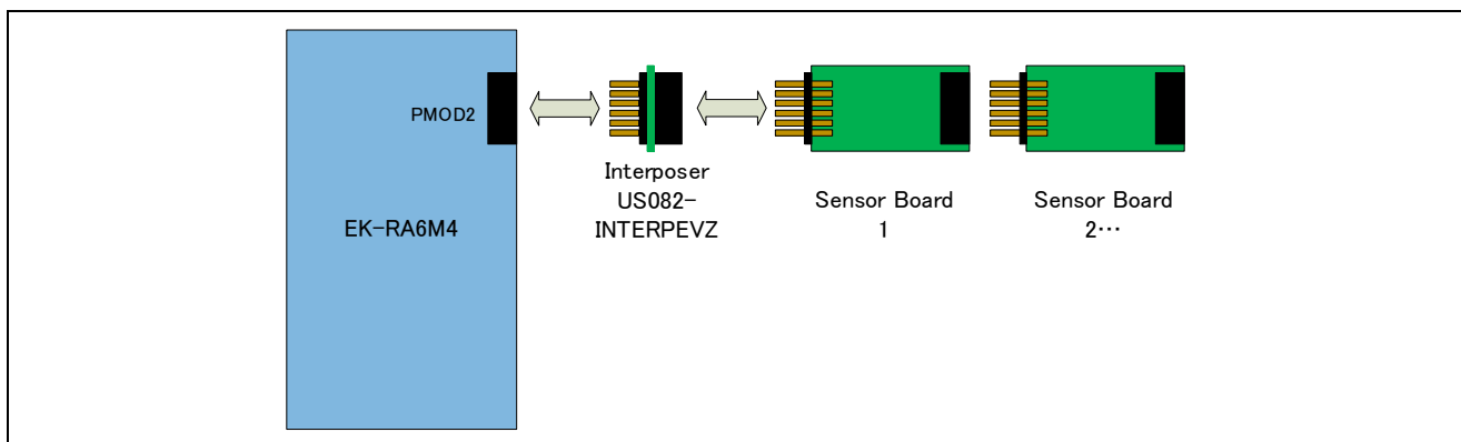
図 2-1 RA HW 接続図
