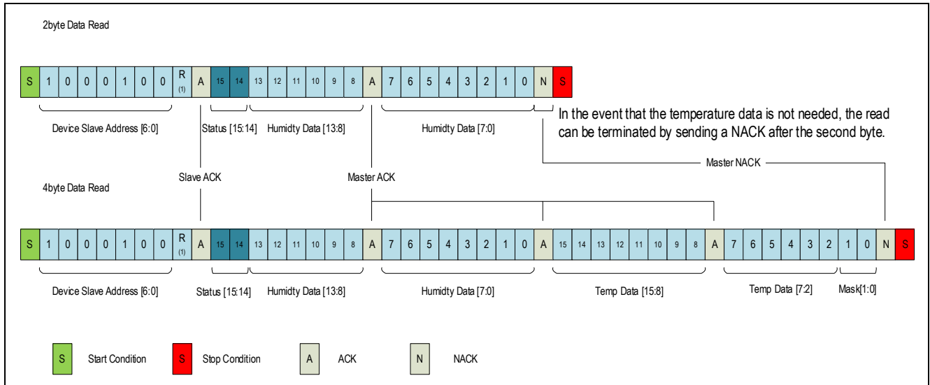
図 3-1 I2C 通信フォーマット
