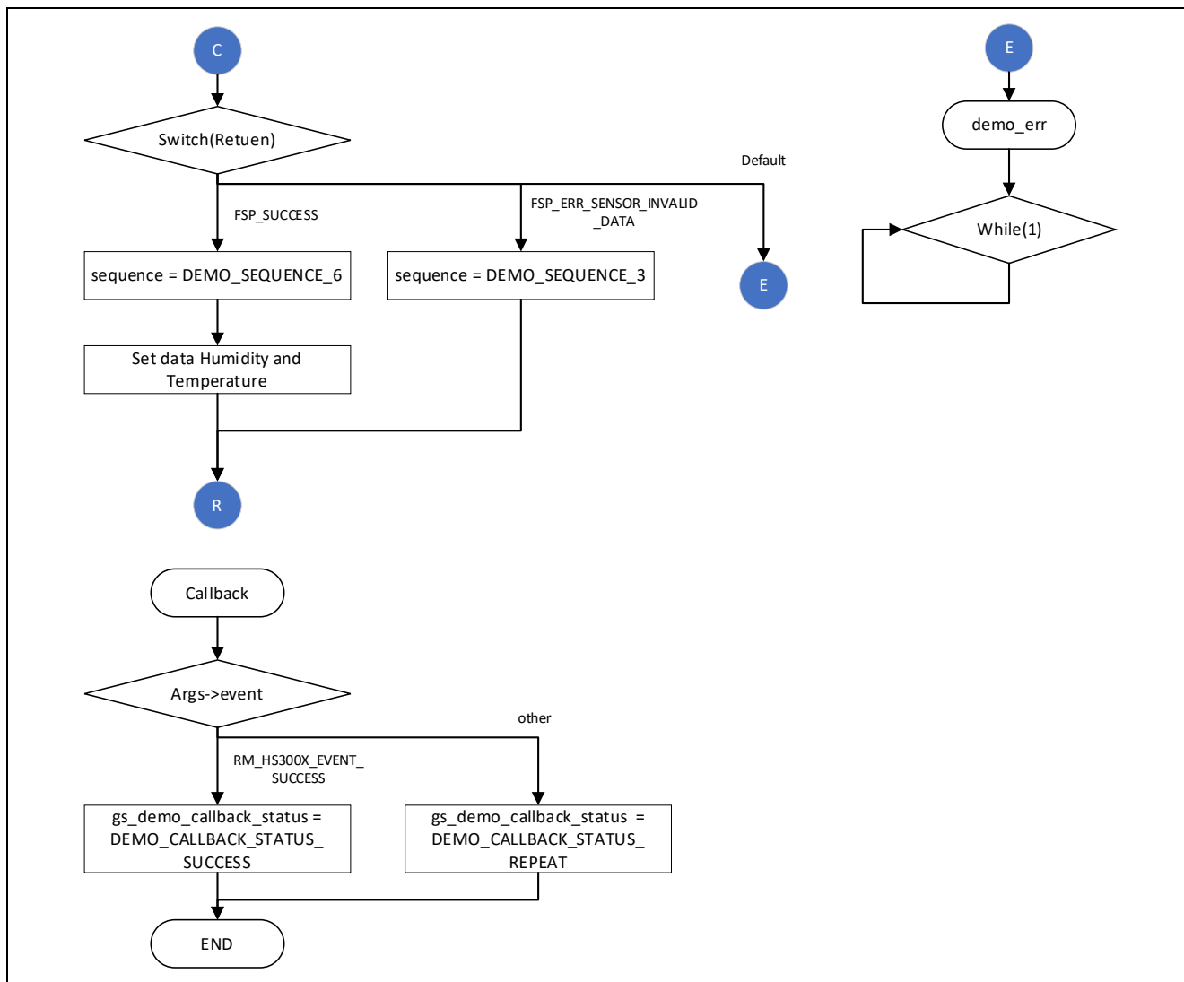
図 4-5 サンプルソフトウェア Non-OS 版メイン処理フロー2
