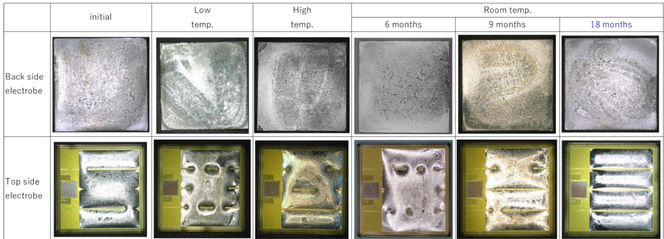
図 4 半田付け後の電極 事例
