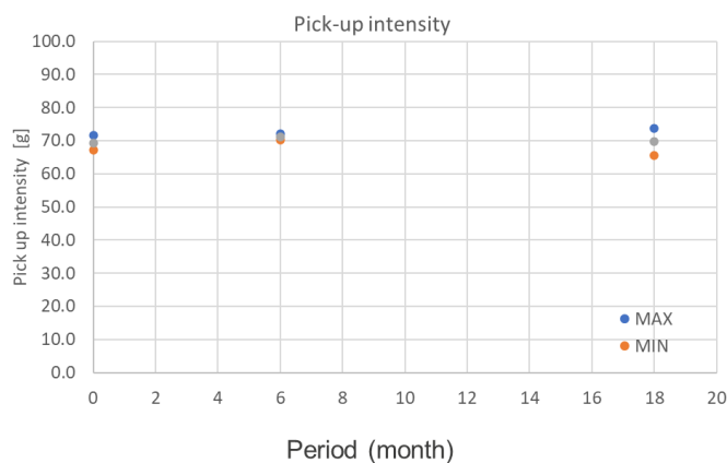
図 5 ピックアップ力 測定結果
