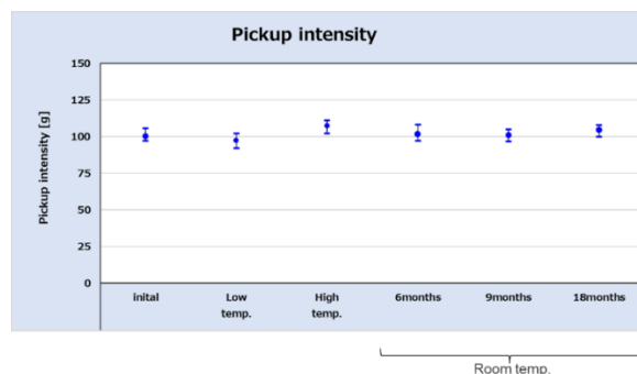
図 3 ピックアップ力 測定結果
