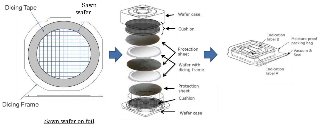
図 1 ウエハ品の梱包仕様例
