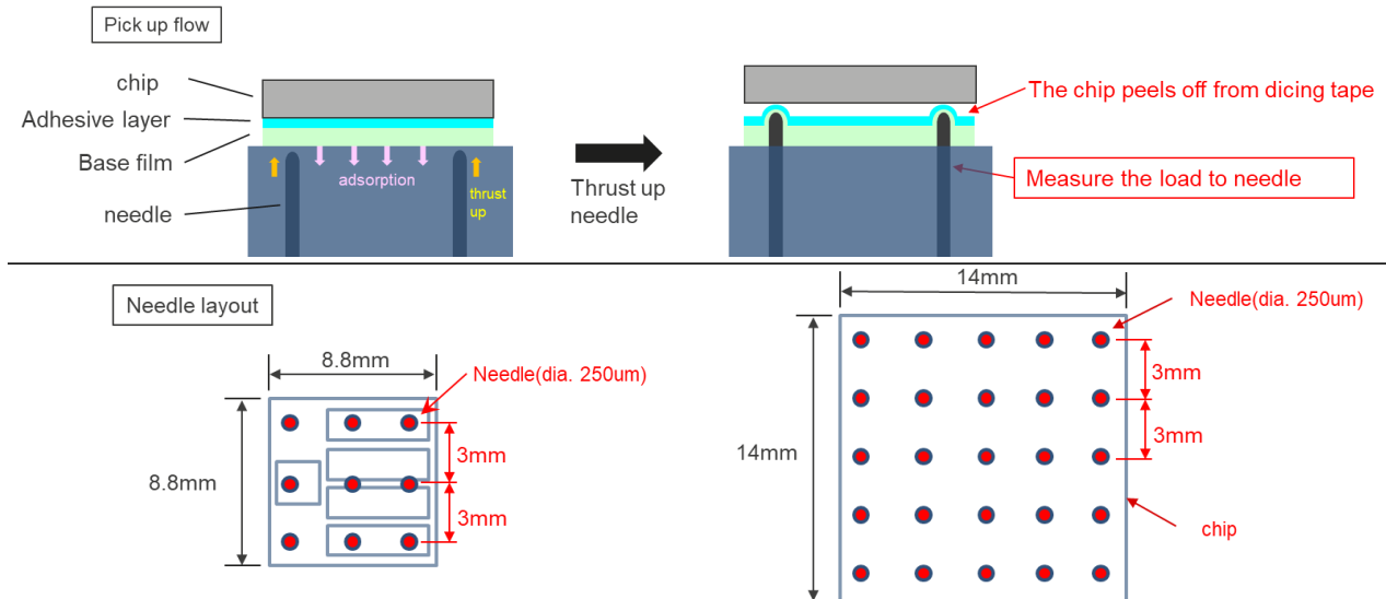
図 2 ピックアップ力の測定方法
