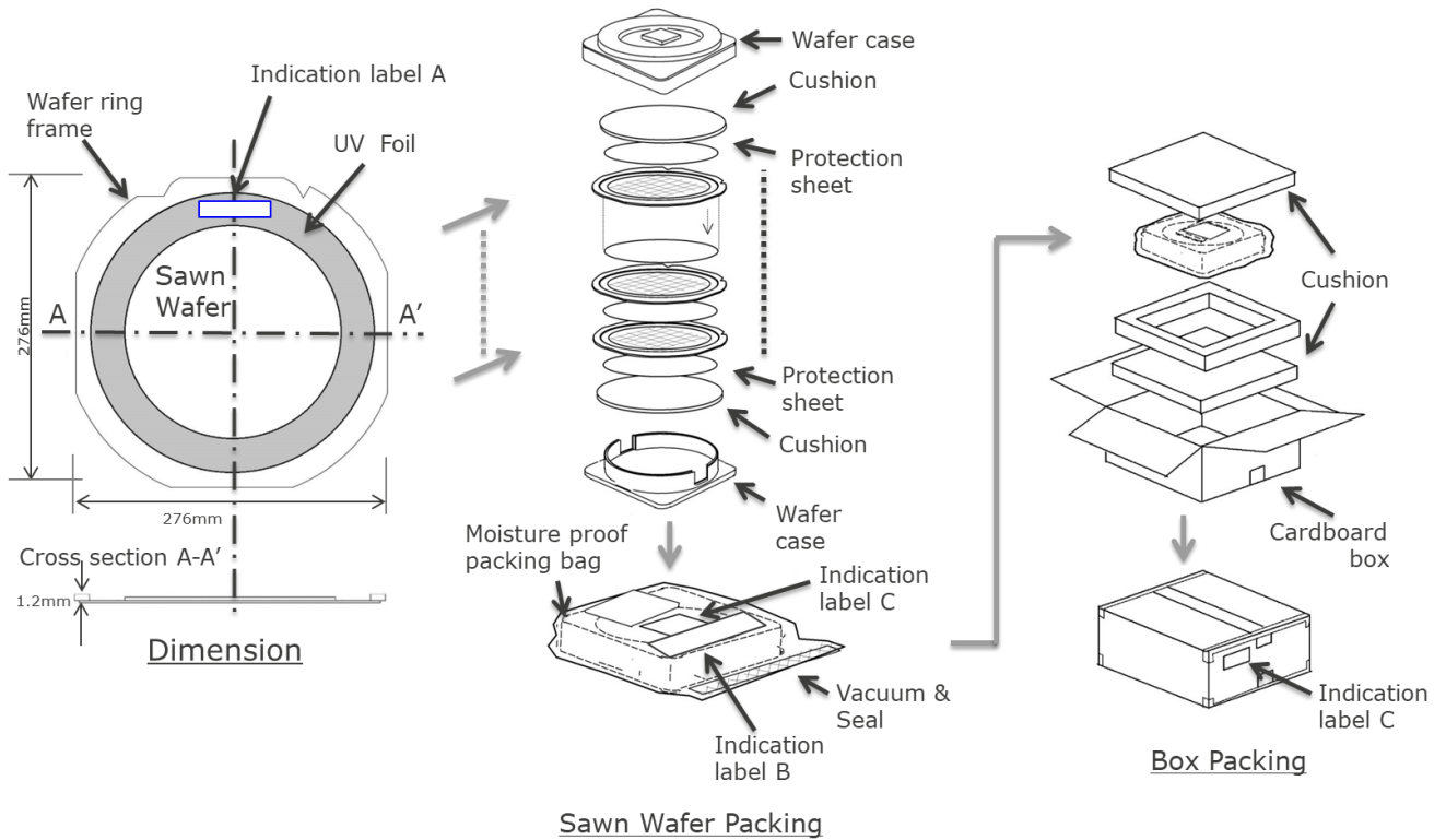
図 1 Sawn Wafer 梱包仕様
