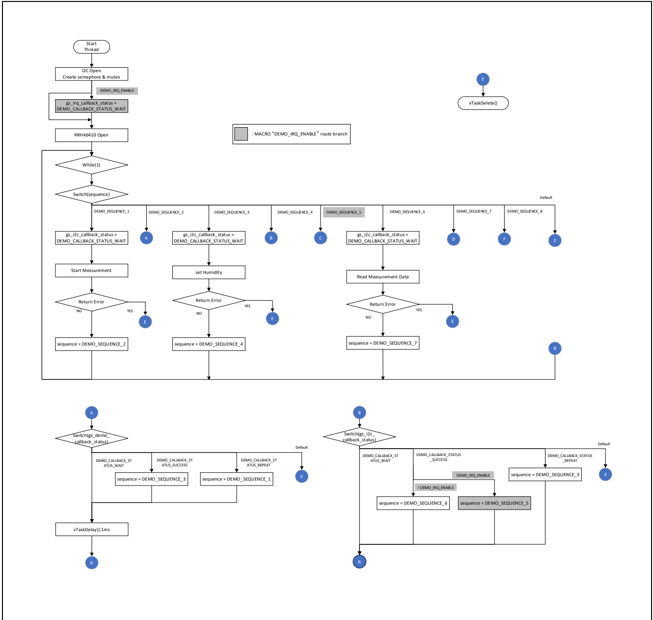
図 4-5 RRH46410 サンプルソフトウェア OS 版メイン処理フロー1
