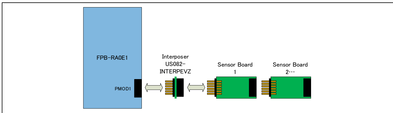
図 2-3 FPB-RA0E1 の Pmod1 Type 2A/Type 3A で IICA を使用した場合の接続図
