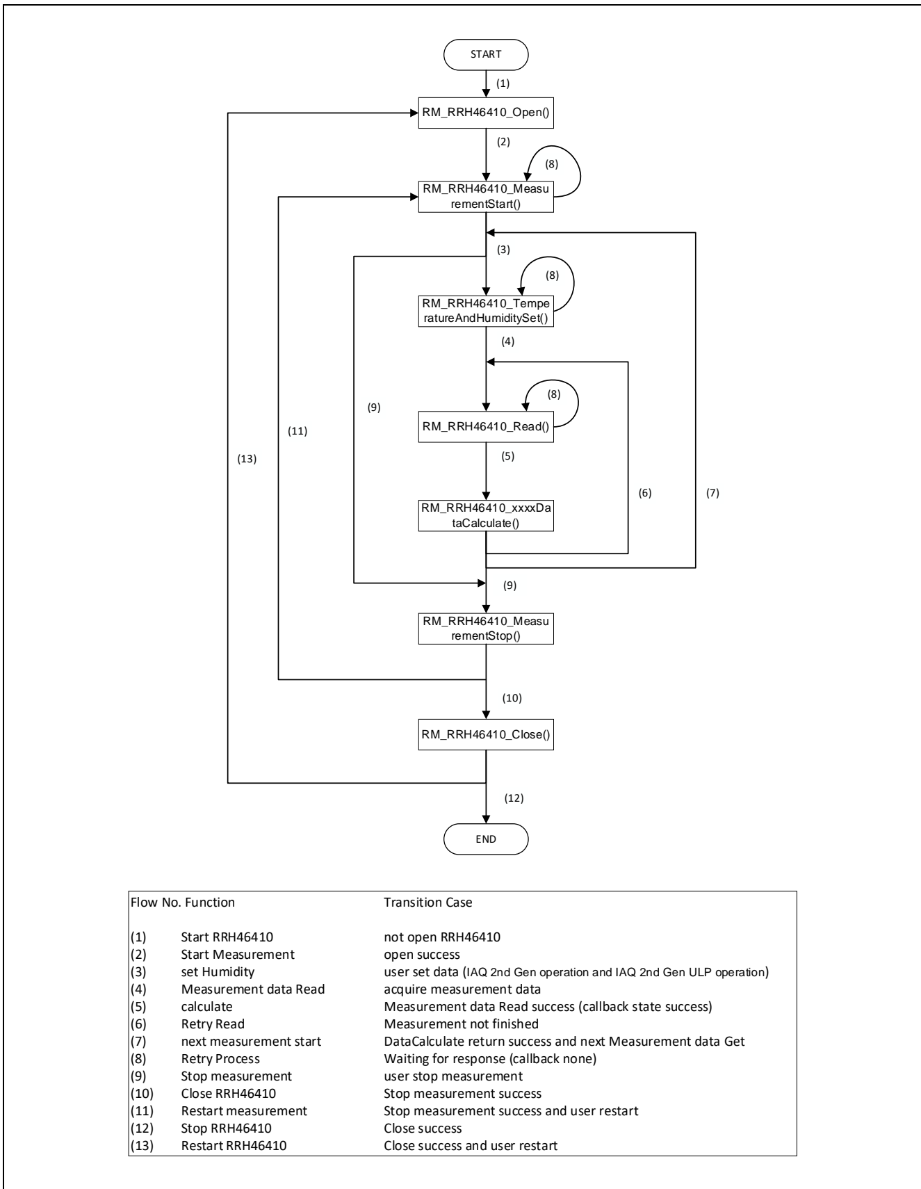
図 4-2 関数 API 遷移図
