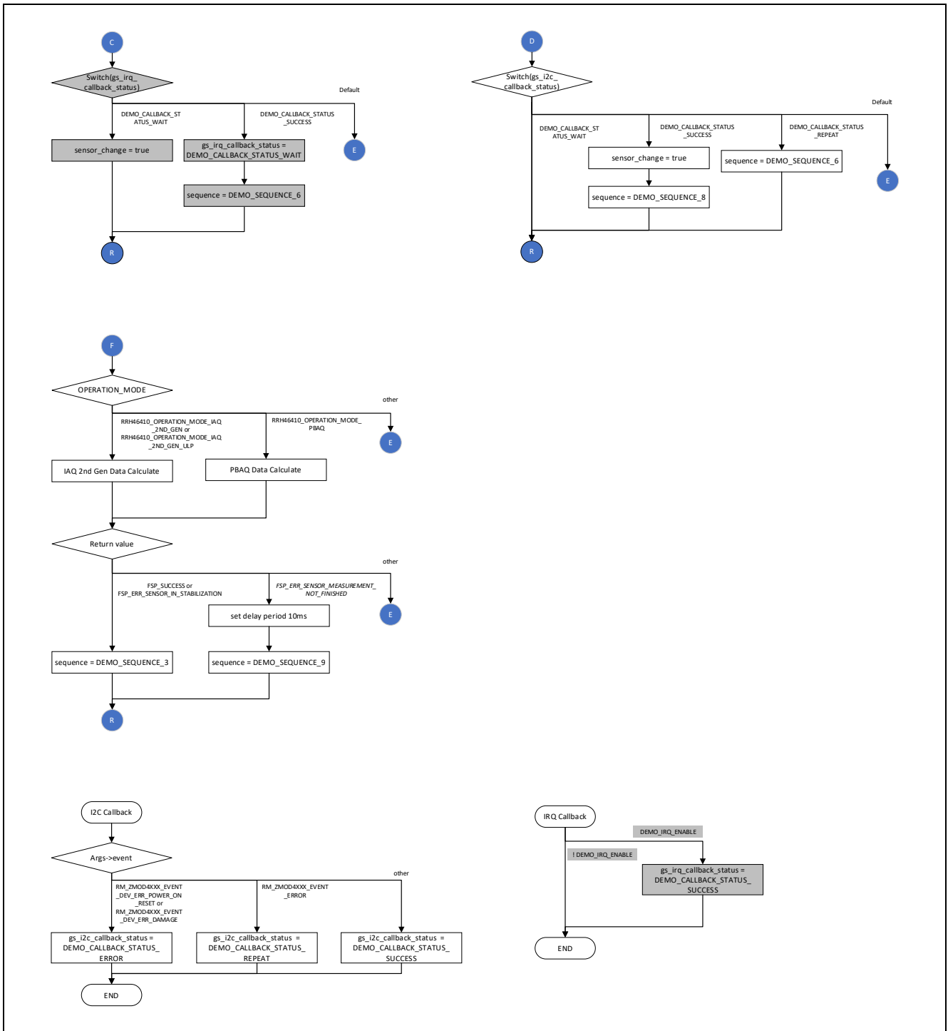
図 4-4 RRH46410 サンプルソフトウェア Non-OS 版メイン処理フロー2
