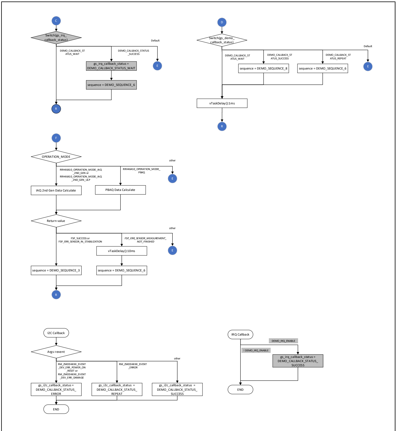
図 4-6 RRH46410 サンプルソフトウェア Non-OS 版メイン処理フロー2
