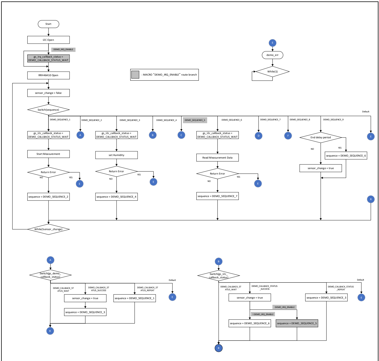
図 4-3 RRH46410 サンプルソフトウェア Non-OS 版メイン処理フロー1
