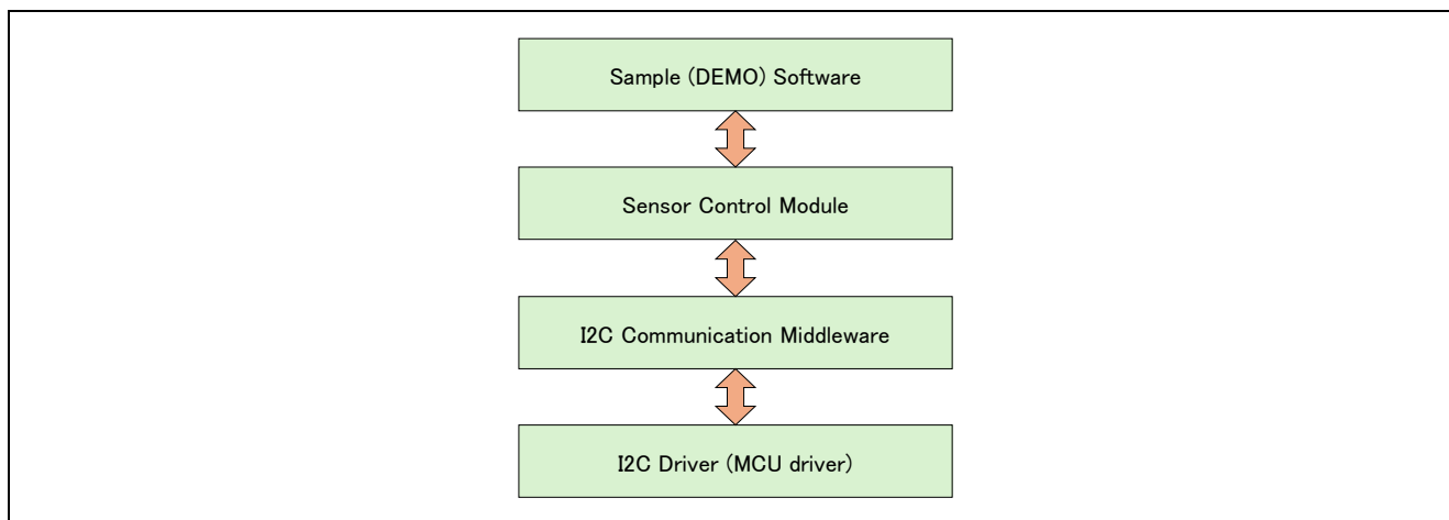
図 4-1 ソフトウェアのレイヤ図
