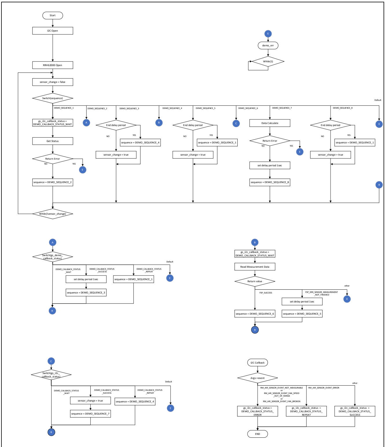
図 4-3 RRH62000 サンプルソフトウェア Non-OS 版メイン処理フロー
