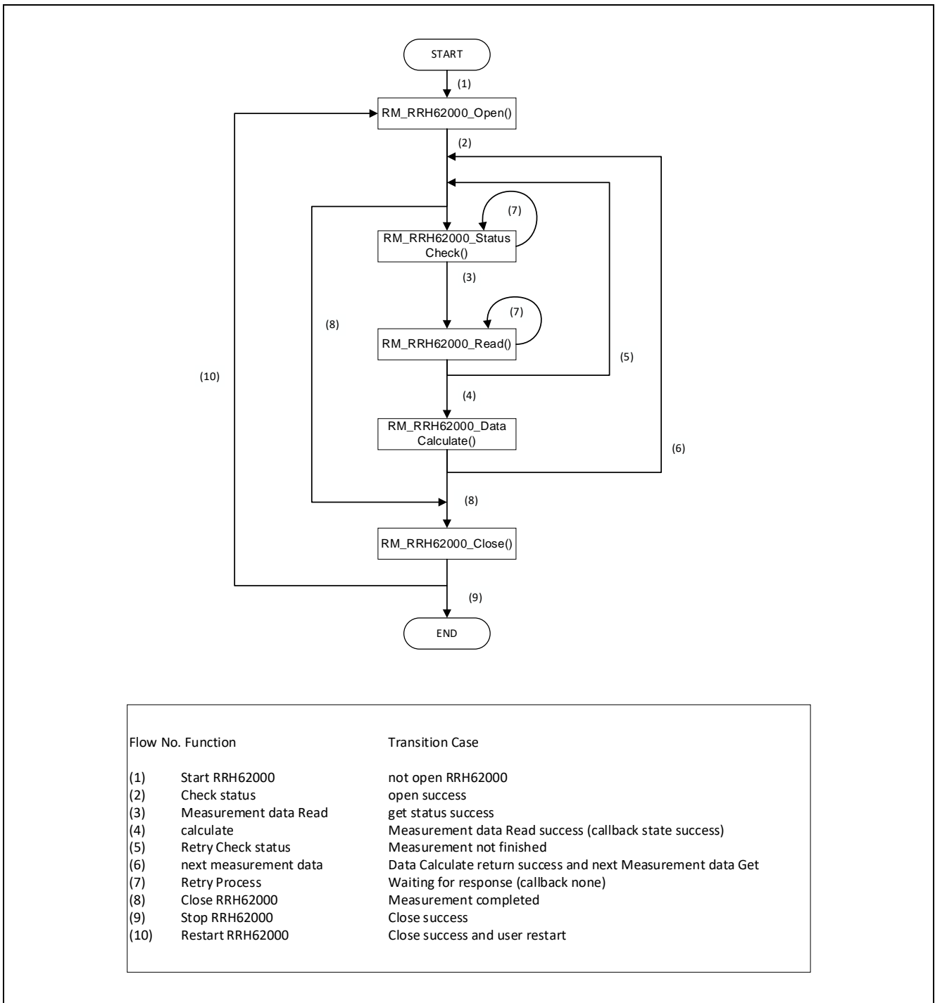
図 4-2 関数 API 遷移図
