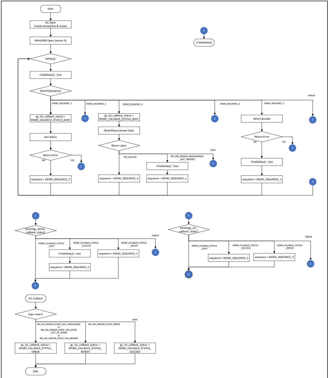
図 4-4 RRH62000 サンプルソフトウェア OS 版メイン処理フロー
