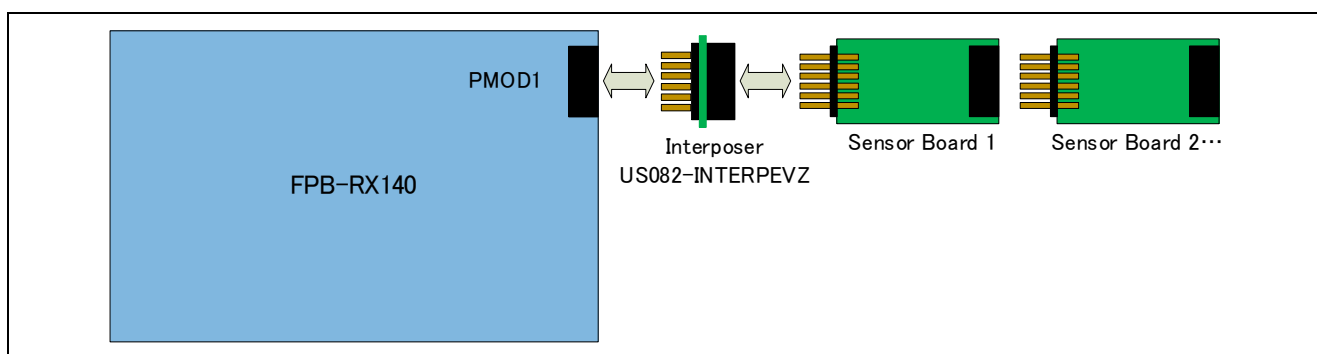
図 2-4 FPB-RX140 HW 接続図
