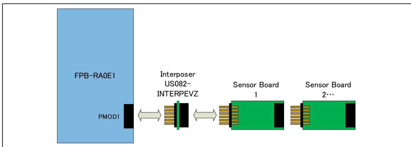
図 2-3 FPB-RA0E1 の Pmod1 Type 2A/Type 3A で IICA を使用した場合の接続図
