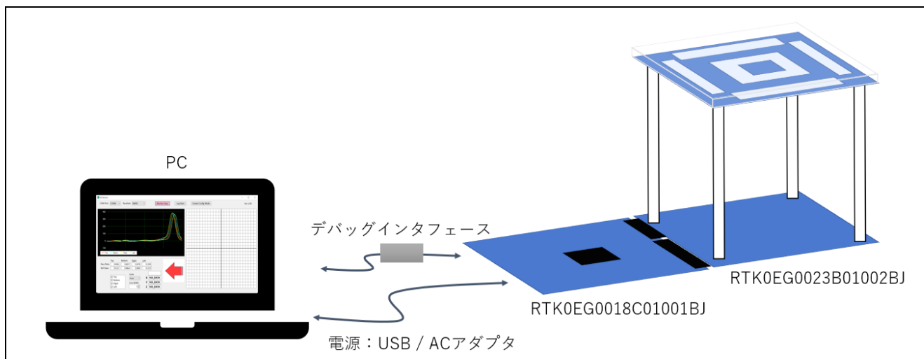
図 2-1 機器接続図
