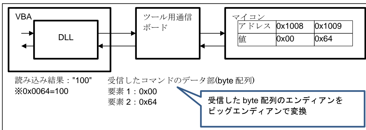
図 5-5 ビッグエンディアン読み込みイメージ
