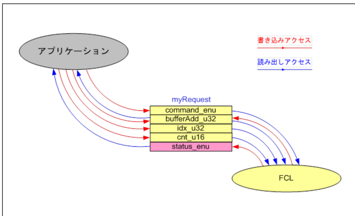
図 3 リクエスト構造体の使用法
