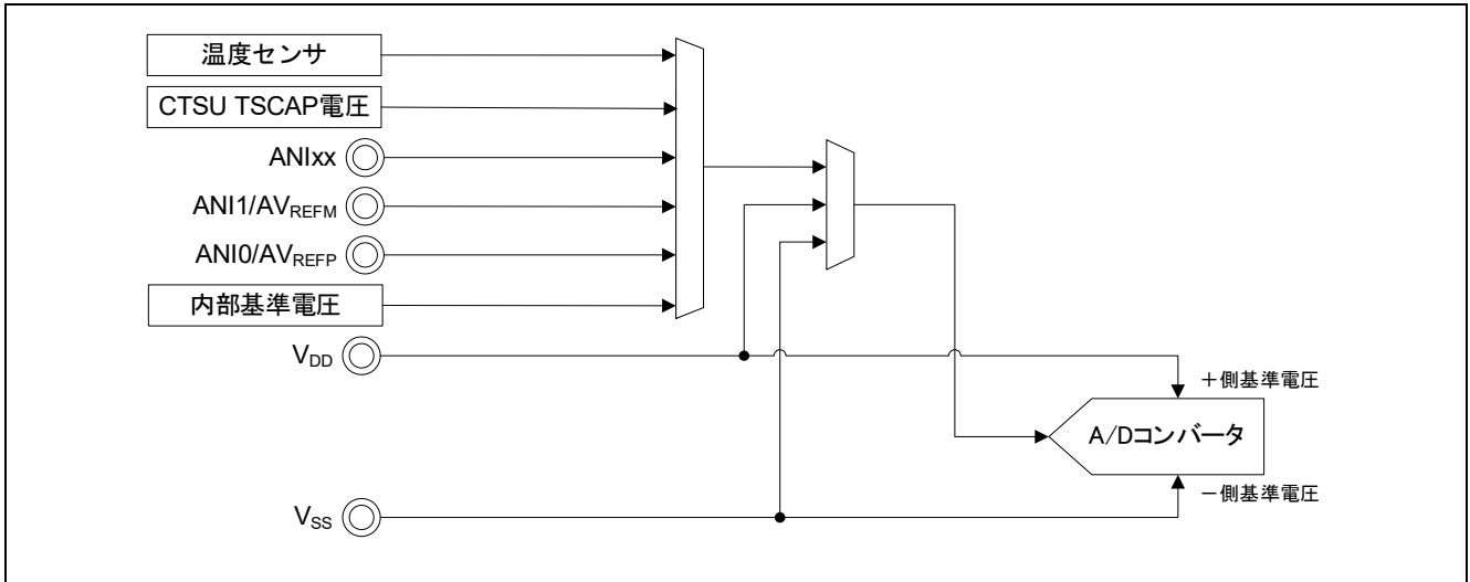
図 2-5 A/D テスト機能の構成 (RL78/G16)
