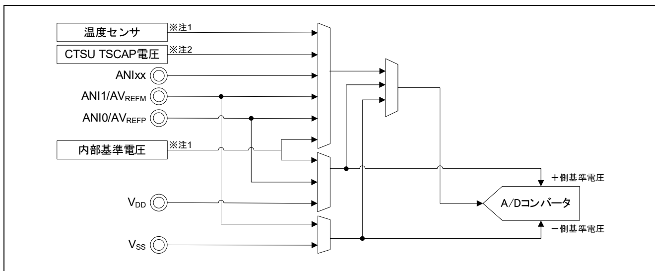
図 2-4 A/D テスト機能の構成 (RL78/G13, G14, G22, G23)
