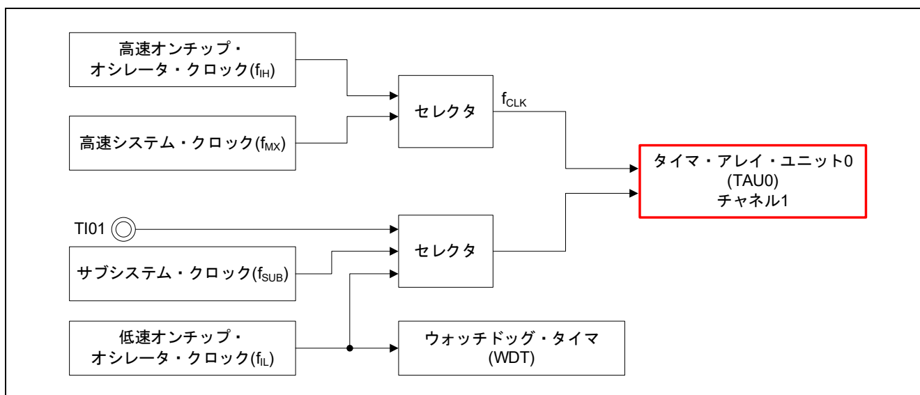
図 2-1 周波数検出機能の構成 (RL78/G14)
