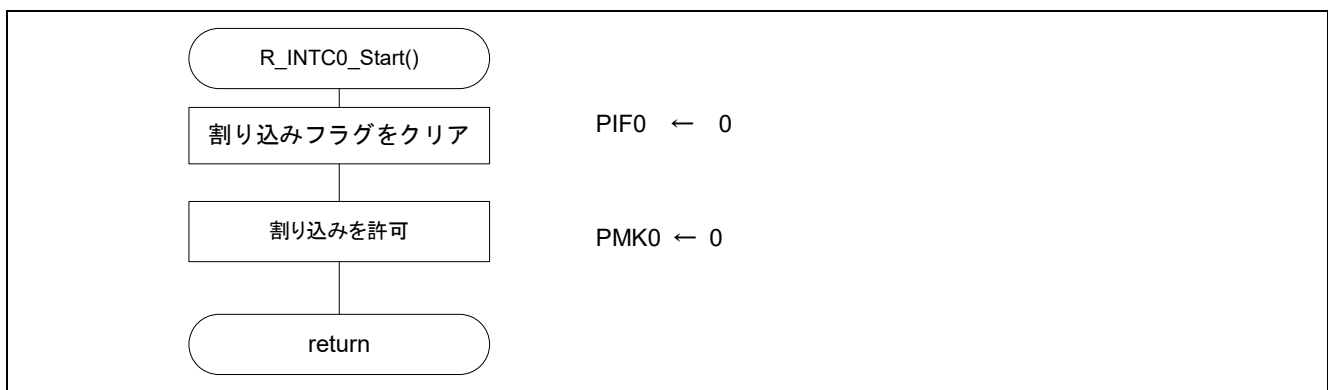
図 4.10 割り込み許可設定
