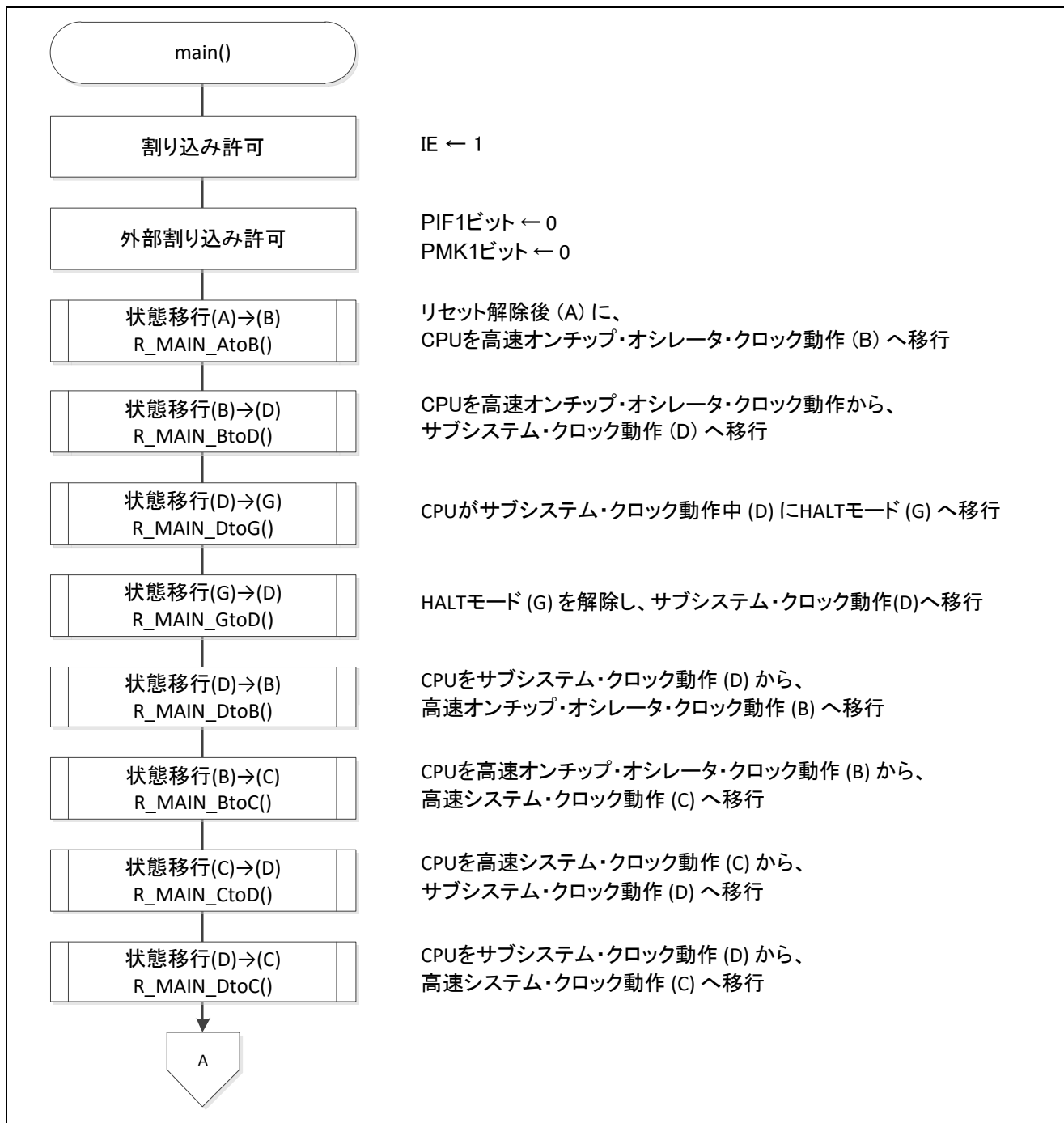
図 5.8 メイン処理(1/2)
