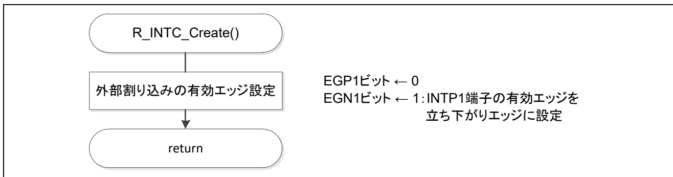
図 5.6 外部割り込みの設定
