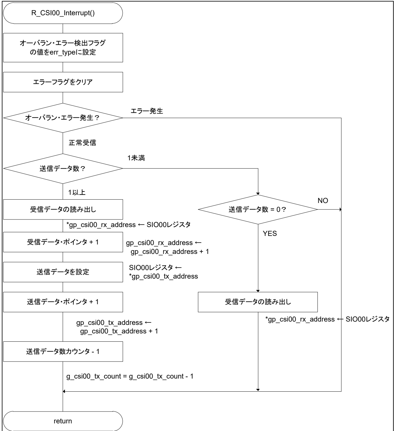
図 5-14 CSI00 の転送完了割り込み処理
