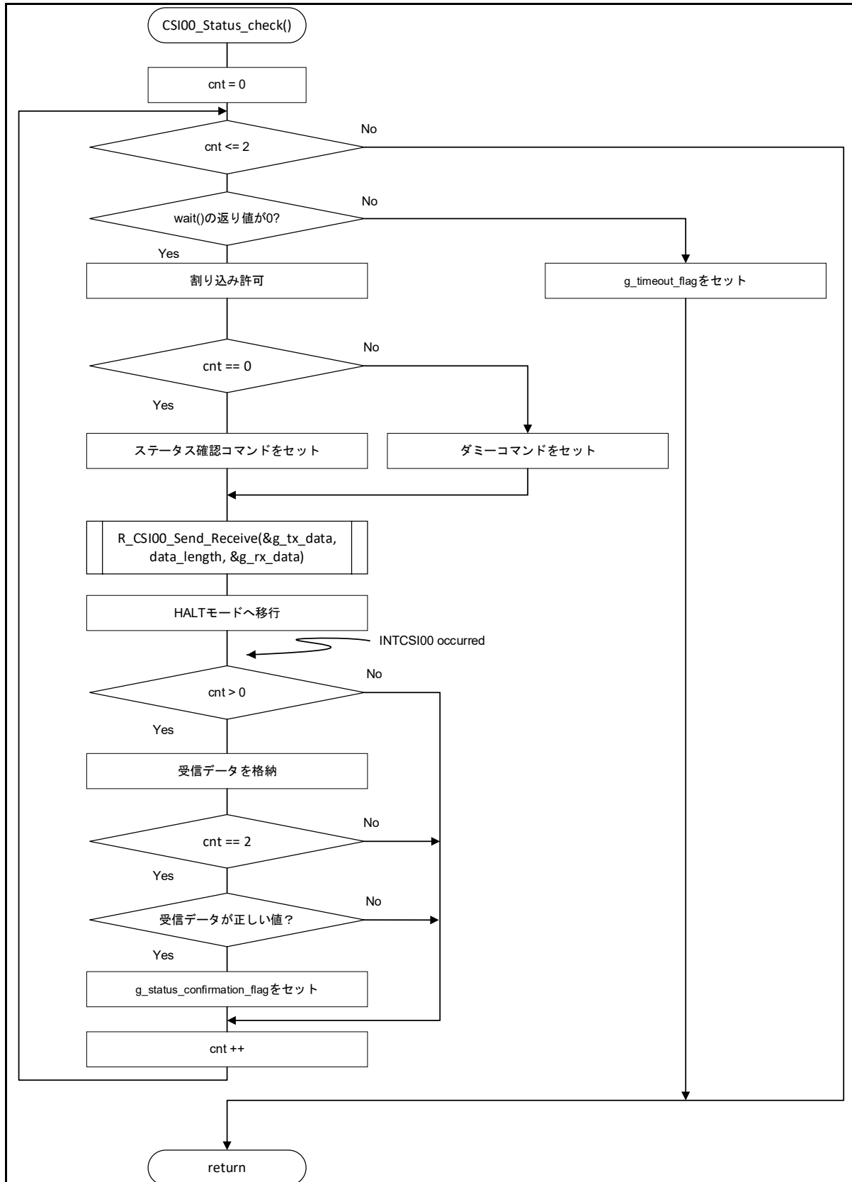
図 5-15 CSI ステータス確認処理
