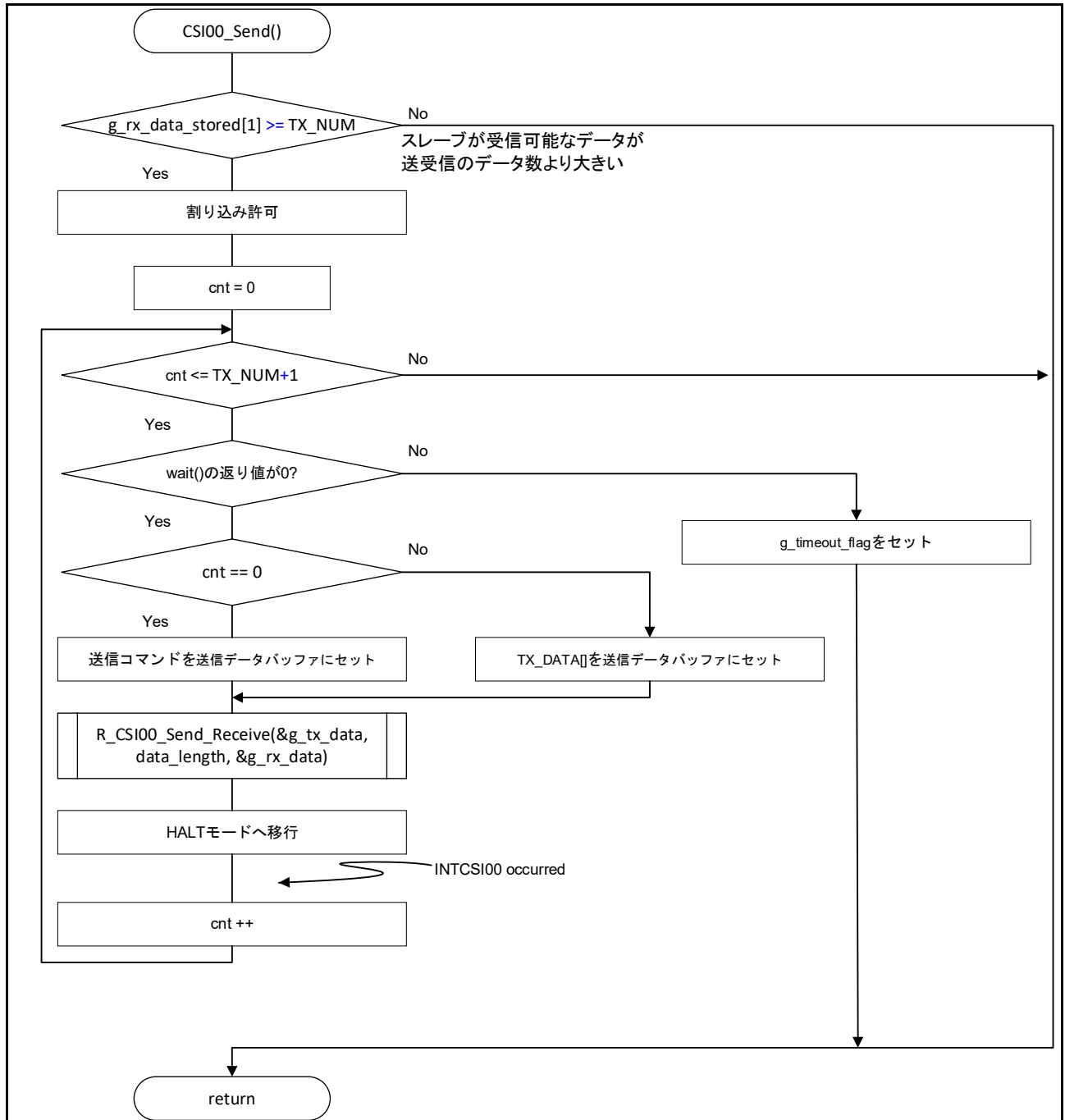
図 5-17 CSI 送信処理
