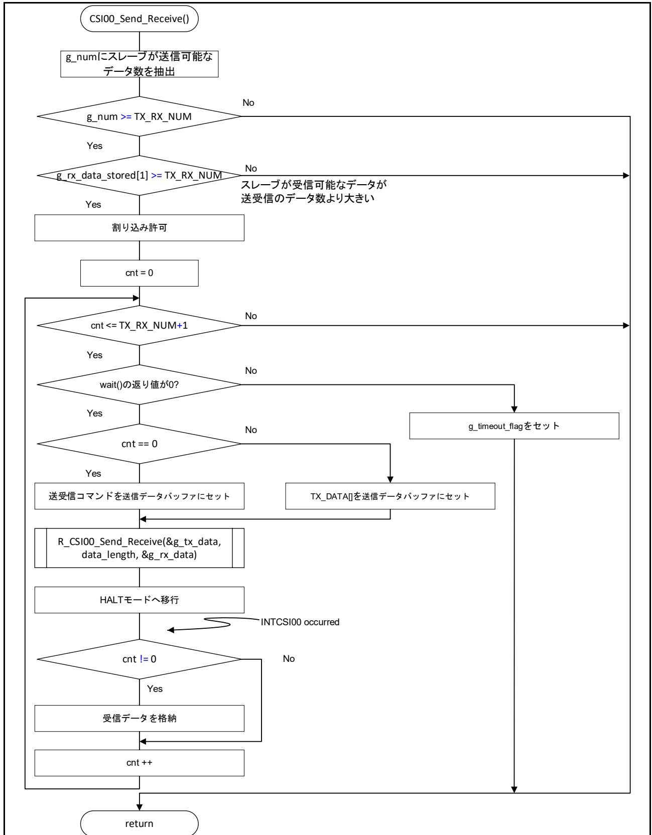
図 5-16 CSI 送受信処理
