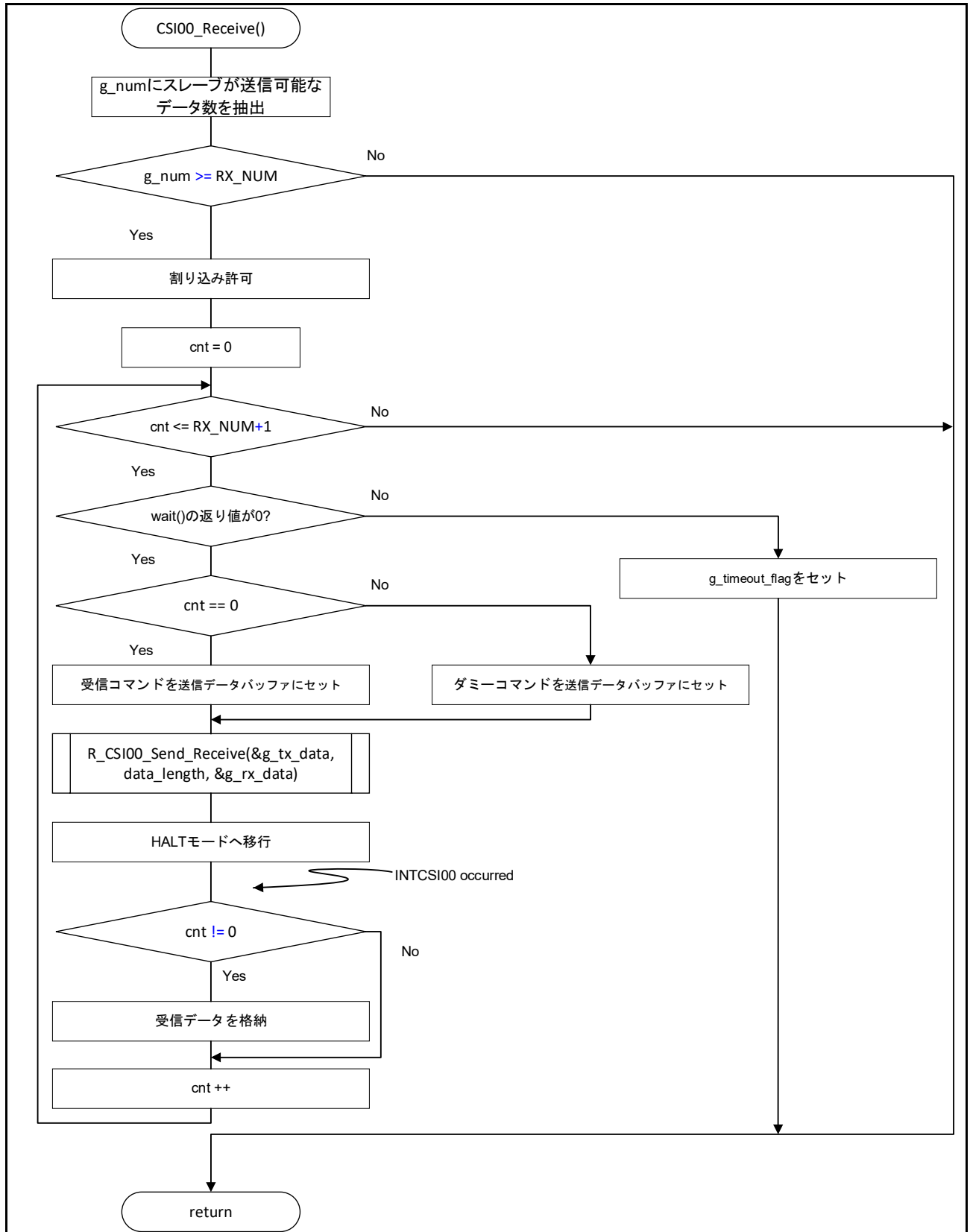
図 5-18 CSI 受信処理
