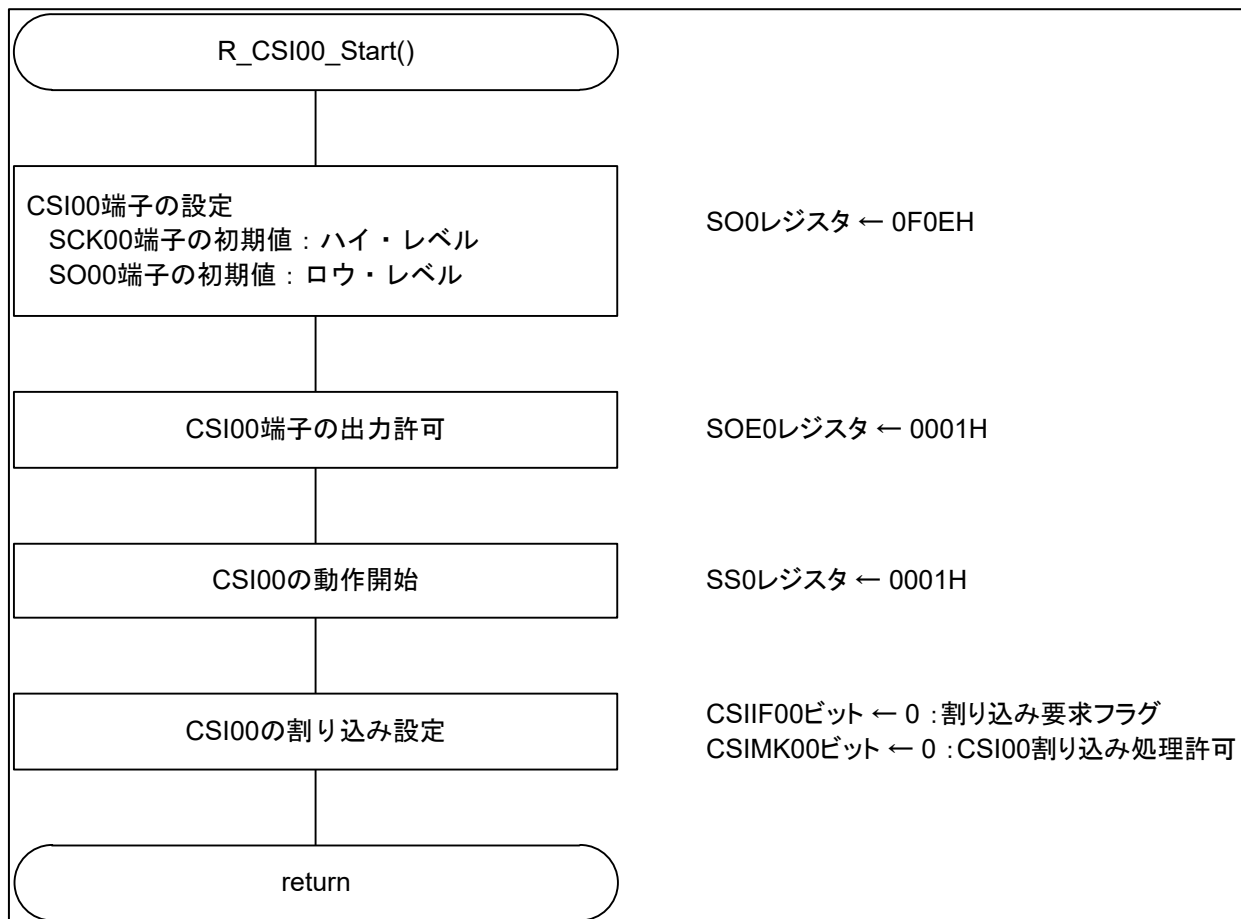
図 5-12 SAU0 チャンネル 0 (CSI00) の動作開始処理
