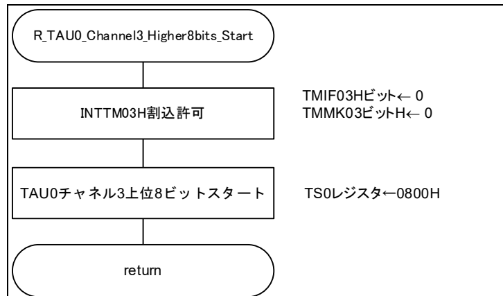
図 5-11 TAU0 チャンネル 3 上位 8 ビット動作開始
