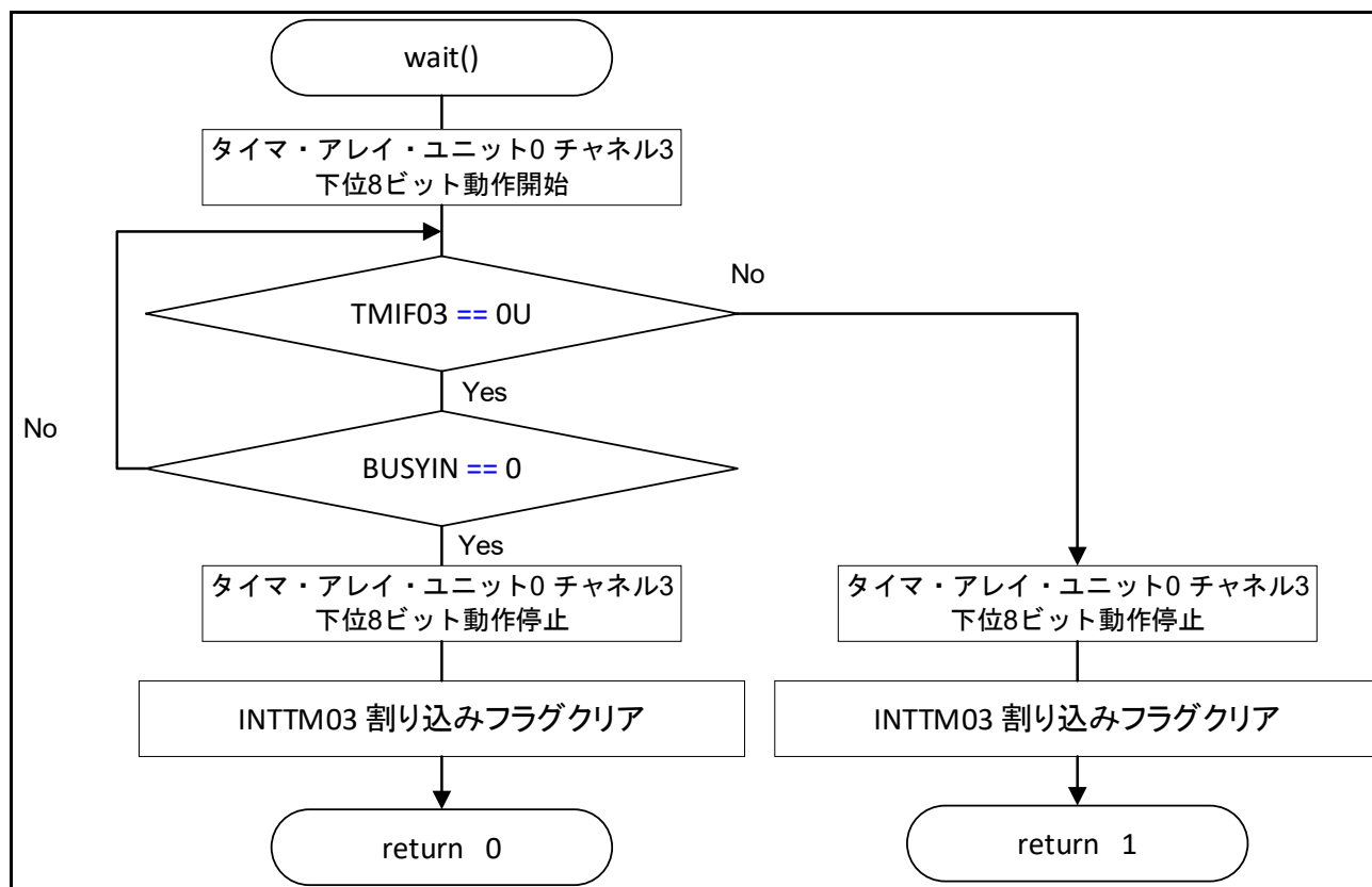
図 5-19 スレーブ応答待ち処理
