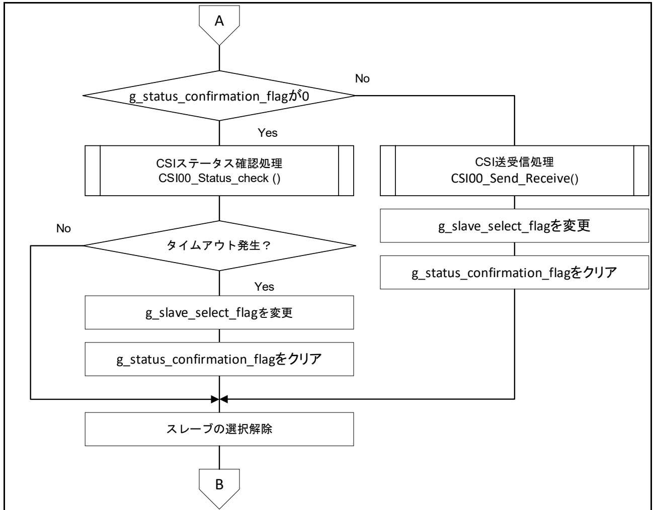
図 5-9 メイン処理 2/2
