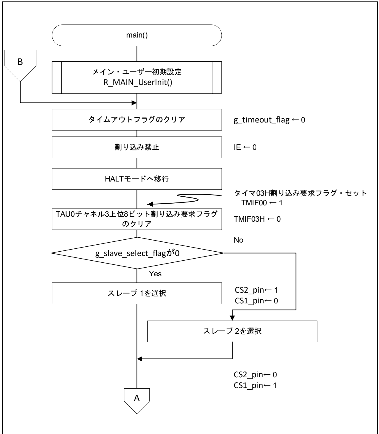
図 5-8 メイン処理 1/2
