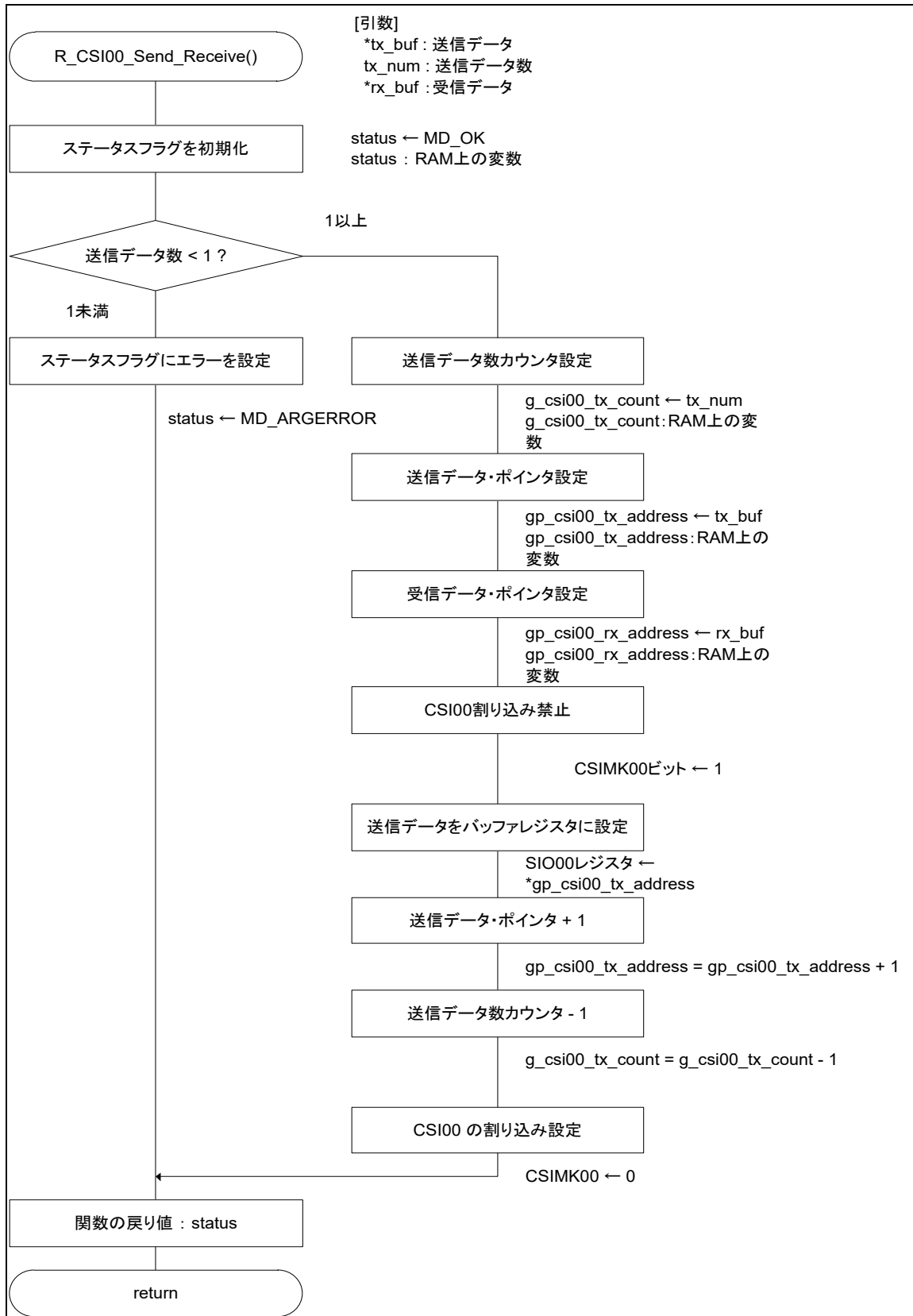
図 5-13 CSI00 データ送受信開始処理
