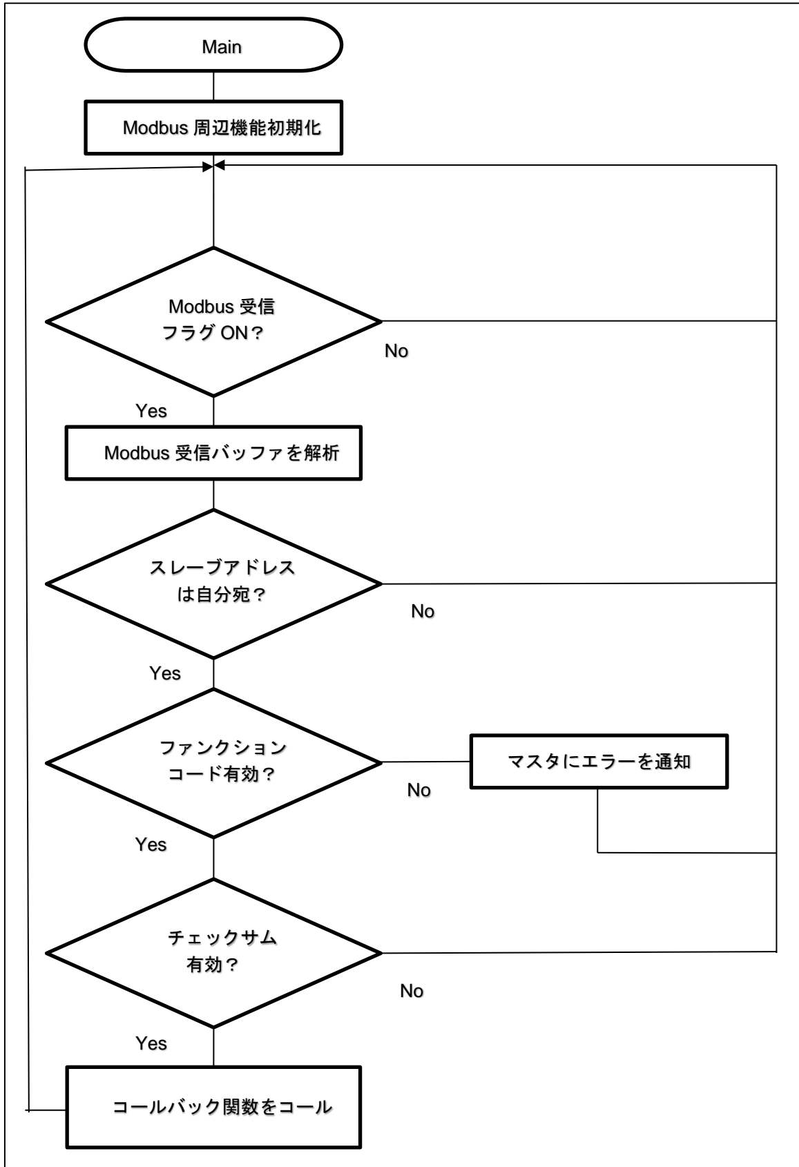
図 5-2 メイン処理（スレーブモード（ASCII））
