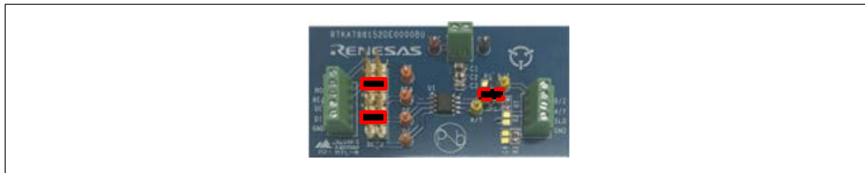
図 4-6 RRTKA788152DE0000BU ジャンパピン接続写真
