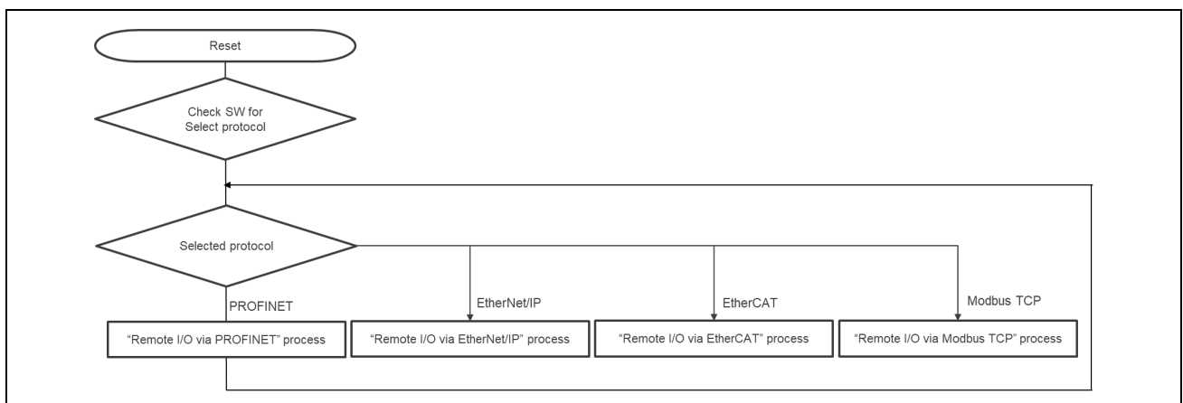
図 3-53 multi-protocol サンプルアプリケーションの流れ
