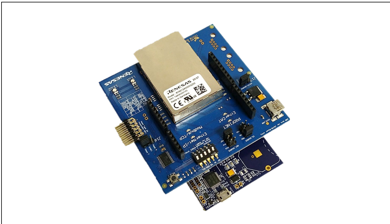
図 1.1 R-IN32M3 モジュール + RL78/G14 Fast Prototyping Board
