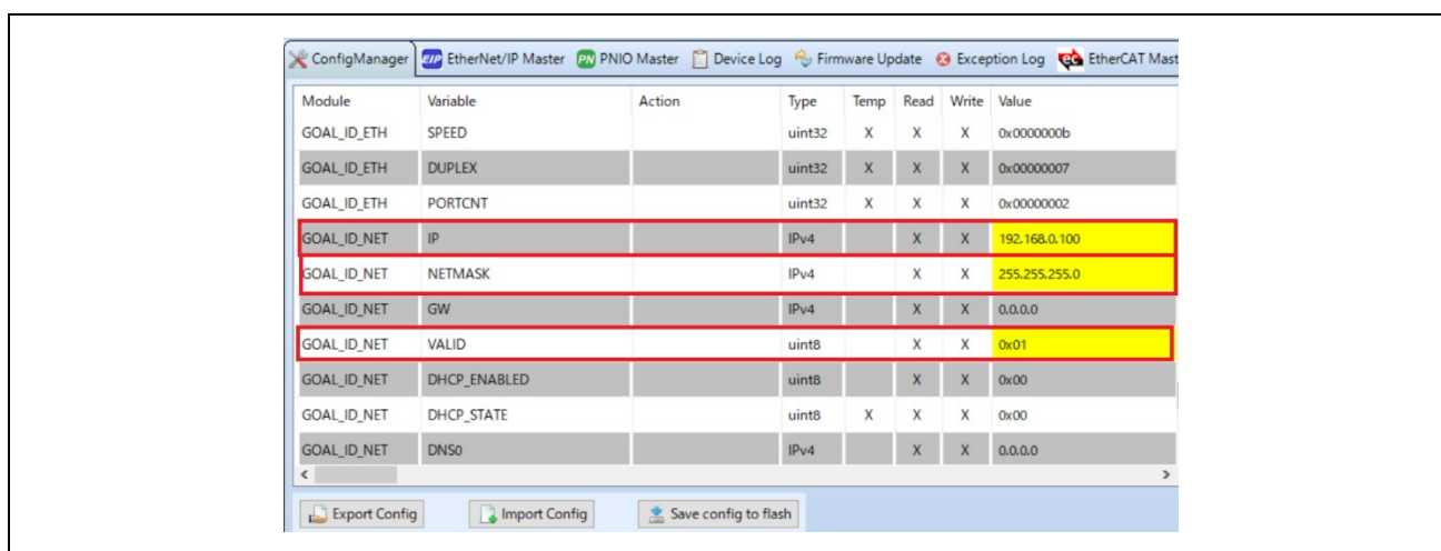
図 3-36 IP アドレス設定
