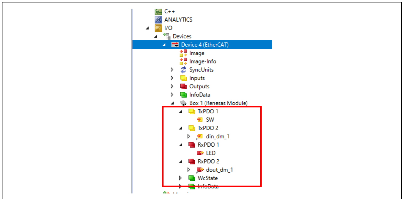
図 3-49 アプリケーション登録 (例 03_ecat)
