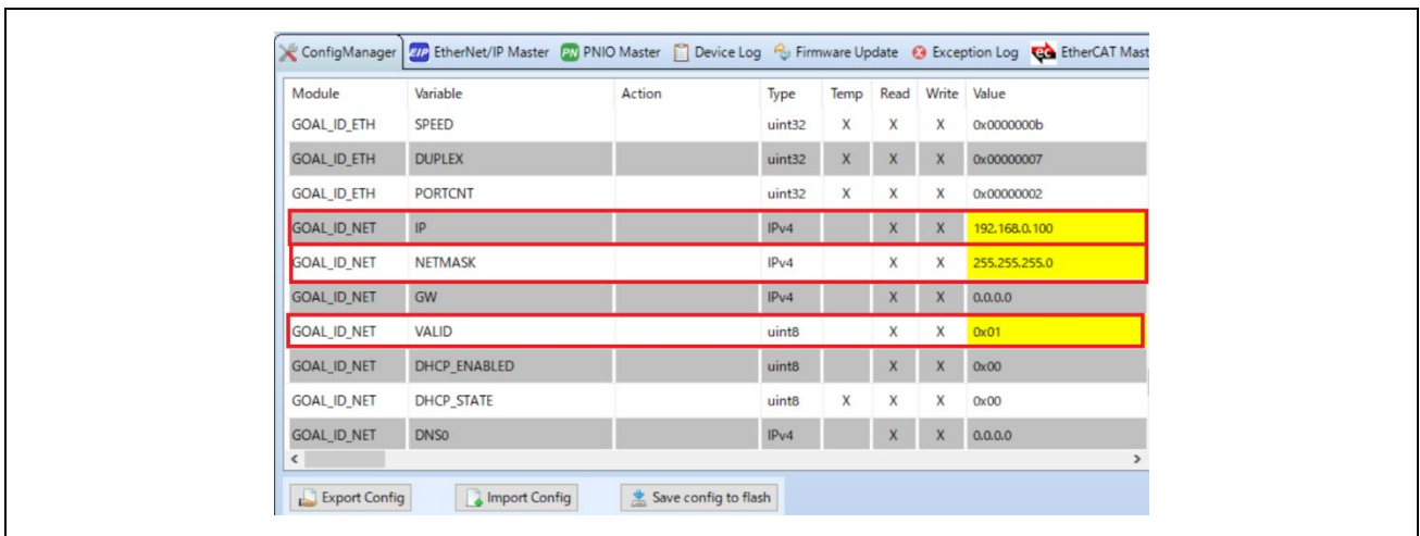
図 3-22 IP アドレス設定
