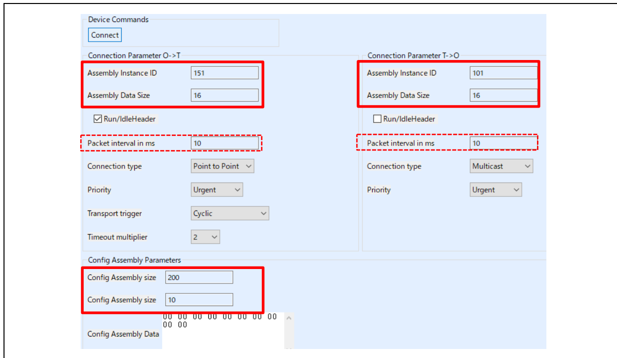
図 3-41 Mirror アプリケーションパラメータ設定
