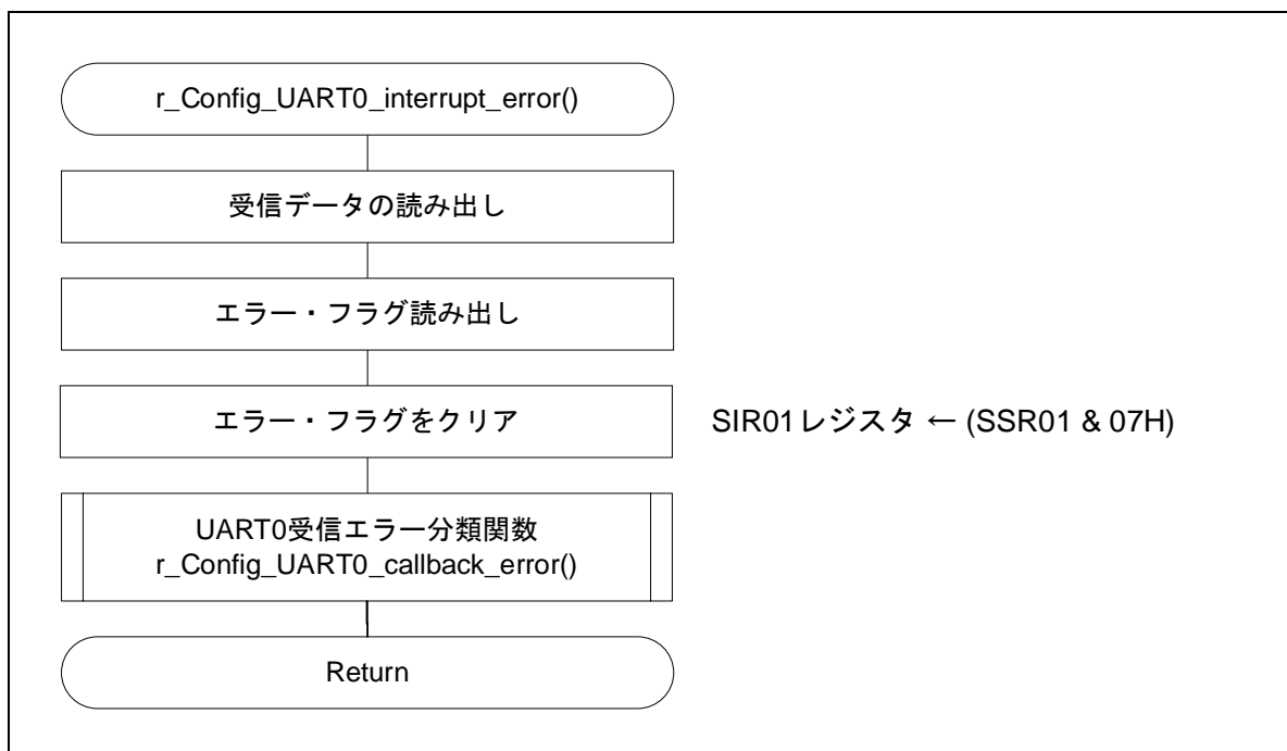
図 4-5 UART0 受信エラー割り込み処理関数
