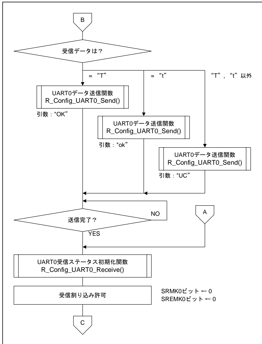
図 4-2 メイン処理 (2/2)
