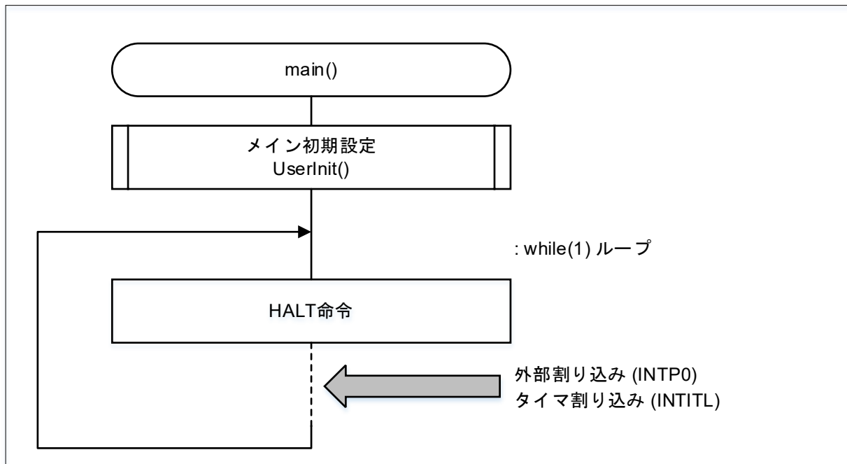
図 4-1 メイン処理
